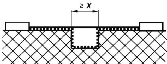
Рисунок F.2 — Широкая канавка
