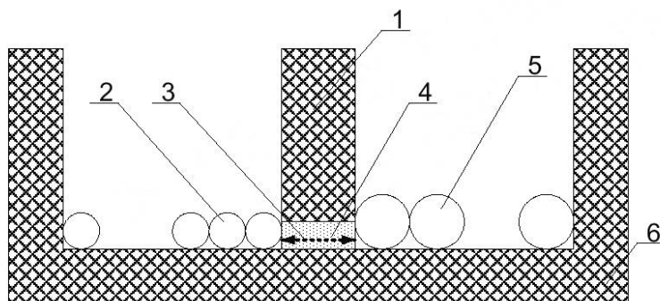
Рисунок F.17 — Компонент, заполненный изоляционным компаундом
