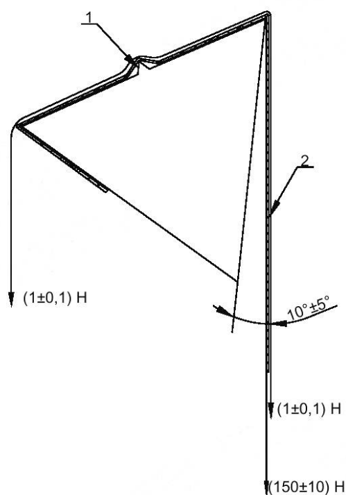
Рисунок AA.2 — Начальное положение оправки
