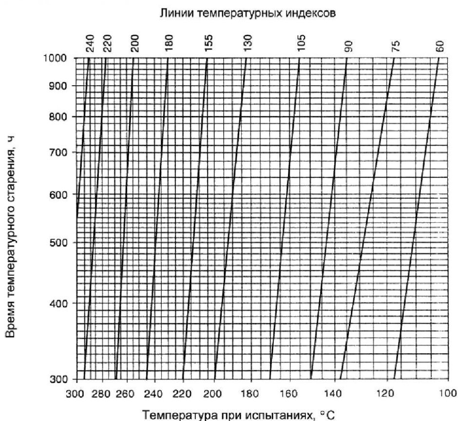
Рисунок 2J — Время теплового старения
