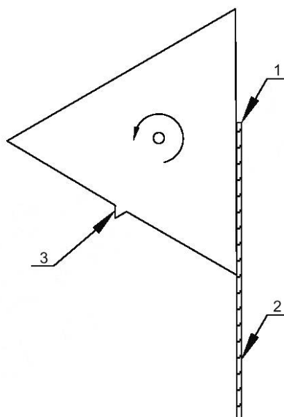
Рисунок AA.2 — Начальное положение оправки
