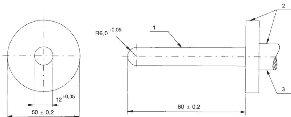
Рисунок 2С — Испытательный щуп
