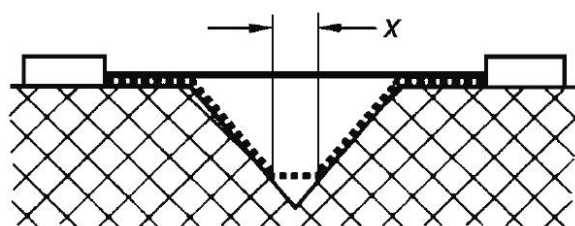
Рисунок F.3 — V-образная канавка
