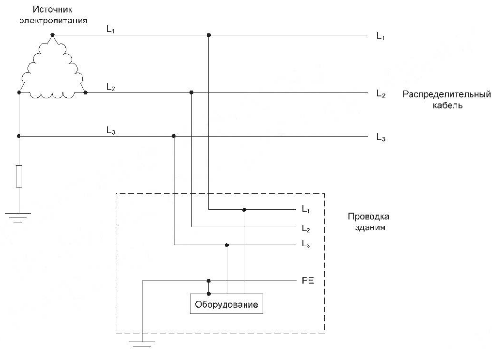
Рисунок V.8 — Пример IT-системы электропитания с тремя фазами
