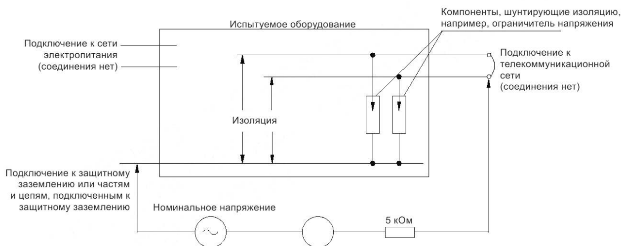
Рисунок 6А — Испытание разделения между телекоммуникационной сетью и землей
