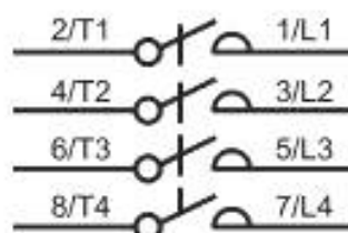
Рисунок А.1 — Клеммы главных цепей
