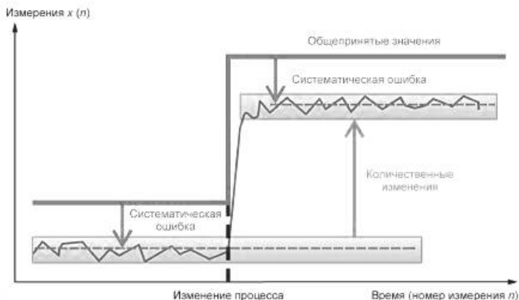
Рисунок О.1 — Пример количественного определения изменения процесса
