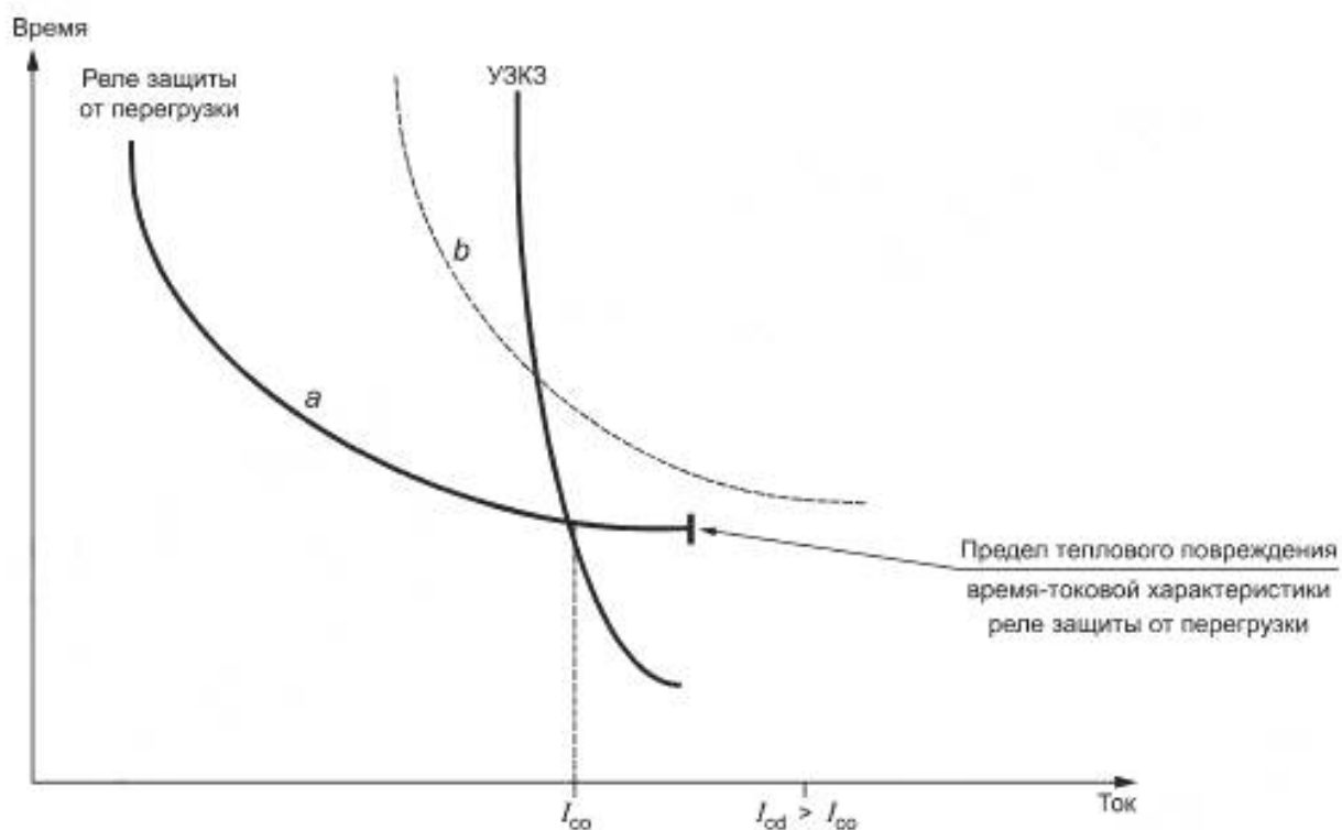
а) Координация с плавким предохранителем
