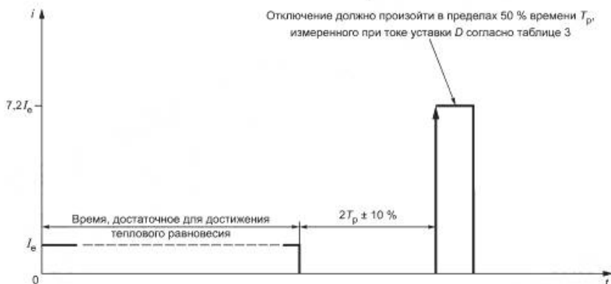
Рисунок 2 — Испытание на проверку тепловой памяти
