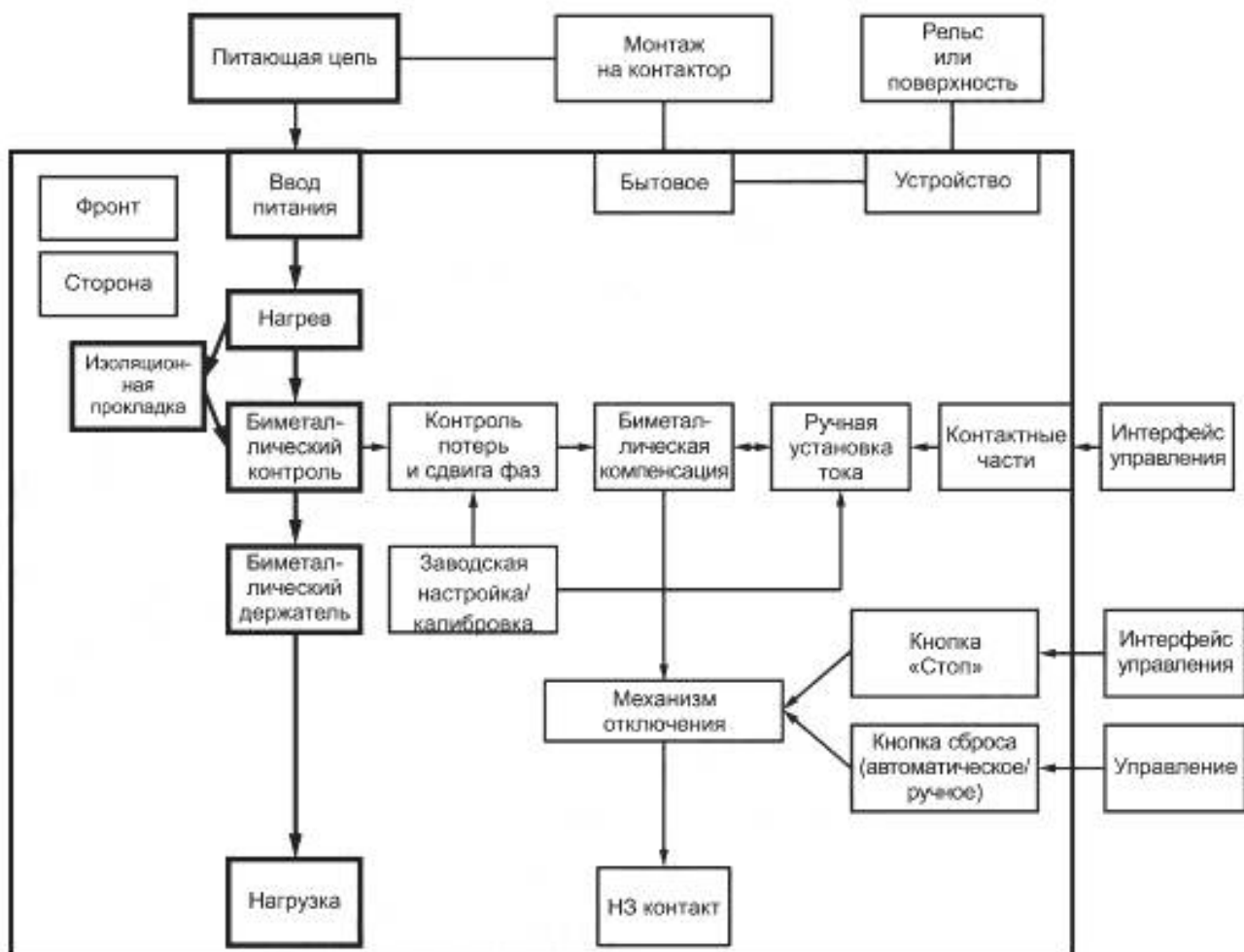
Рисунок L.2 — Типовая конструкция термореле перегрузки
