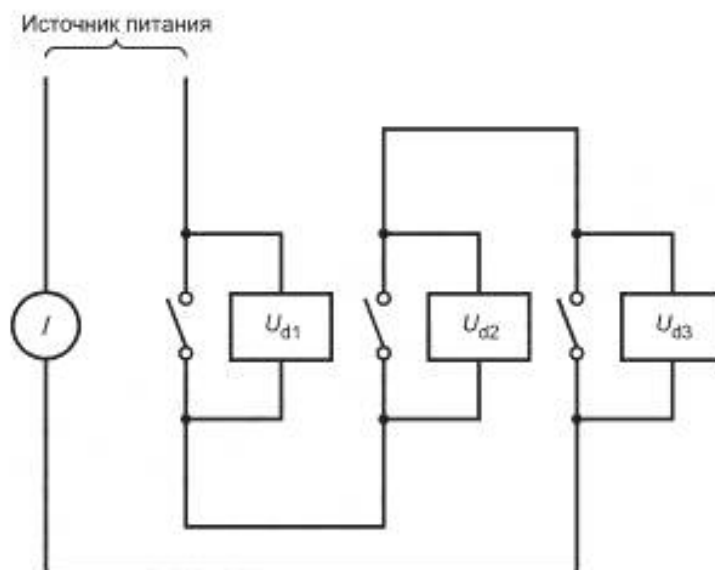
Рисунок 5 — Пример измерения полного сопротивления полюса 3-полюсного контактора
