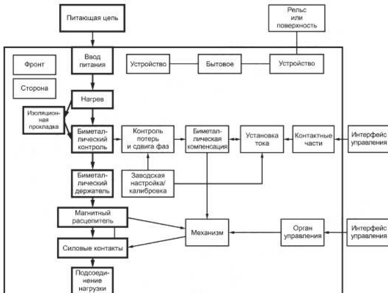
Рисунок L.3 — Типовая конструкция MPSD
