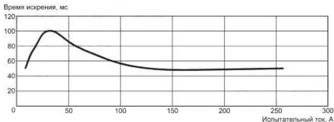
Рисунок М.1 — Критический ток
