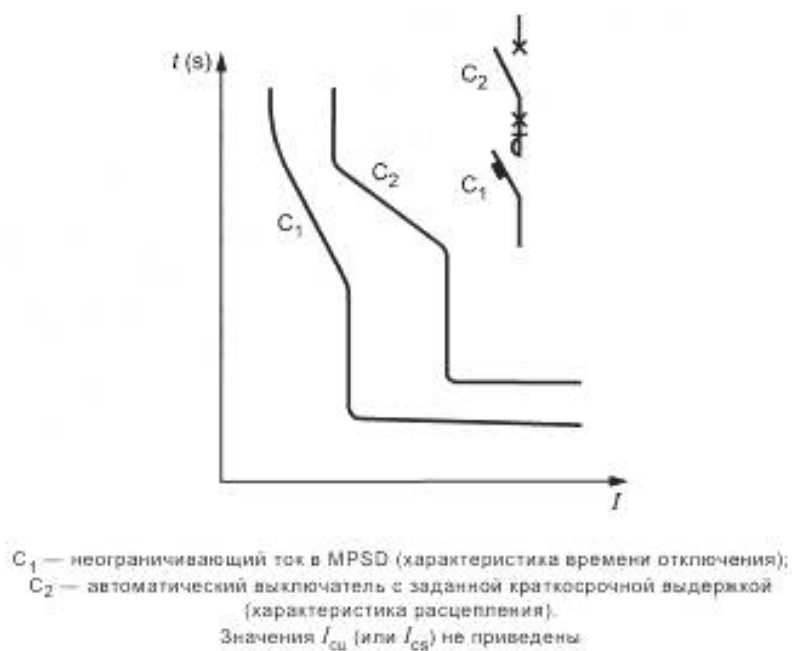
Рисунок Q.3 — Полная селективность между MPSD и автоматическими выключателями. Вариант 2
