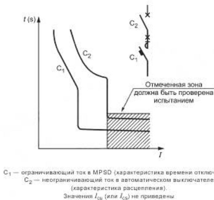
Рисунок Q.2 — Полная селективность между MPSD и автоматическими выключателями. Вариант 1
