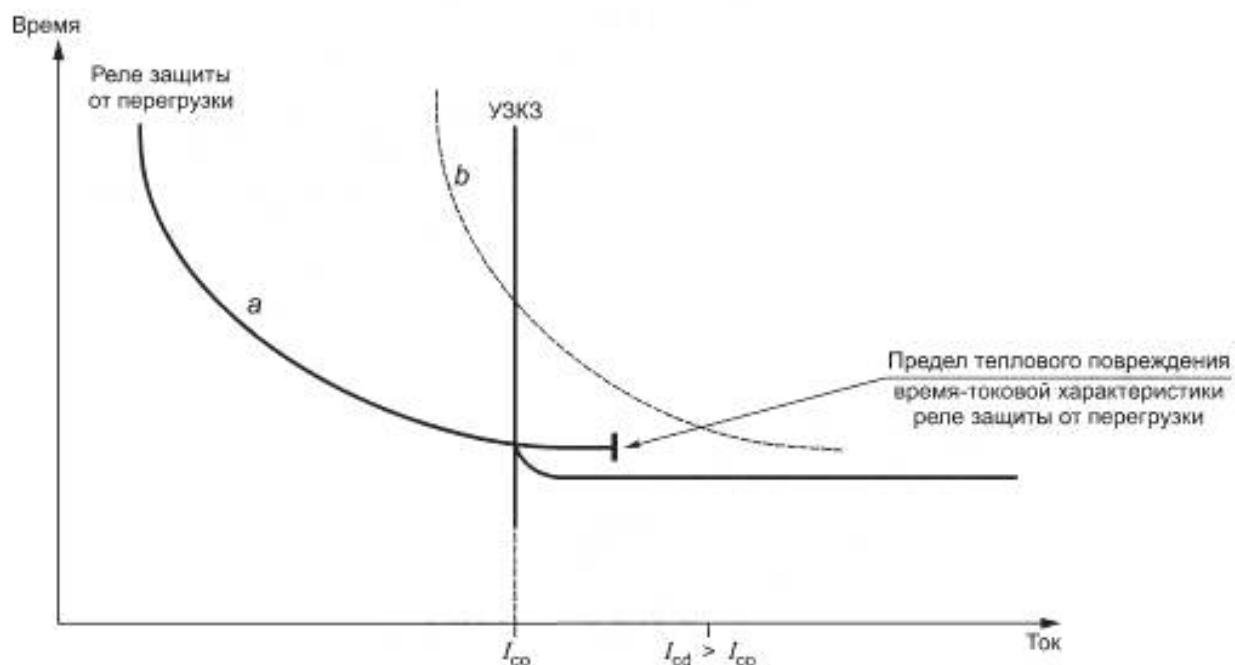
б) Координация с автоматическим выключателем
