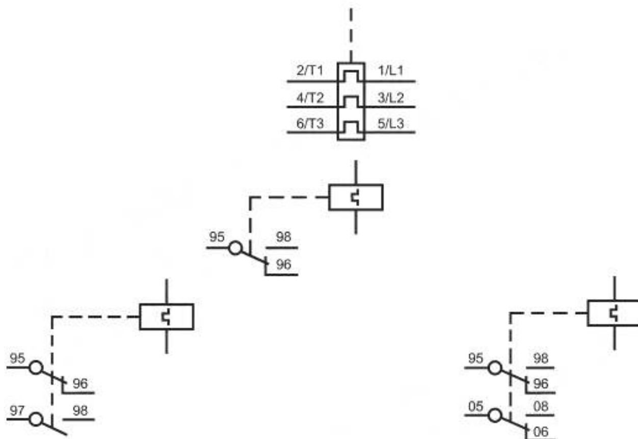
Рисунок А.2 — Реле перегрузки
