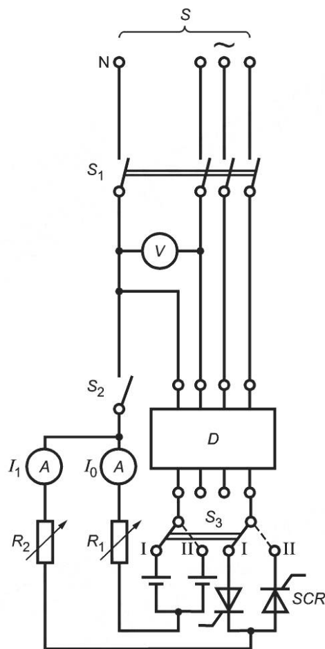
Рисунок В.7 — Пример испытательной цепи для проверки устойчивости к нежелательному отключению в случае искрения без последующего тока (см. В.8.6.3)
