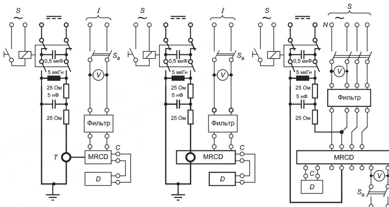
б) Модульное устройство защиты от тока утечки со встроенным сенсорным элементом
