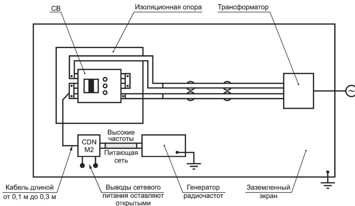
Рисунок F.21 — Схема расположения соединений для проверки устойчивости к кондуктивным помехам, создаваемым полями высокой частоты. Конфигурация двух последовательных фазовых полюсов
