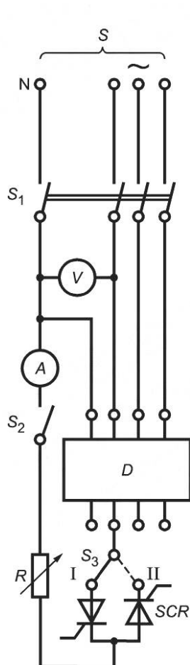
Рисунок В.7 — Пример испытательной цепи для проверки устойчивости к нежелательному отключению в случае искрения без последующего тока (см. В.8.6.3)
