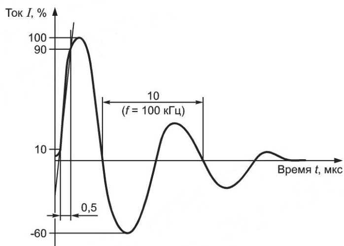
Рисунок В.4 — Волна тока 0,5 мкс/100 кГц
