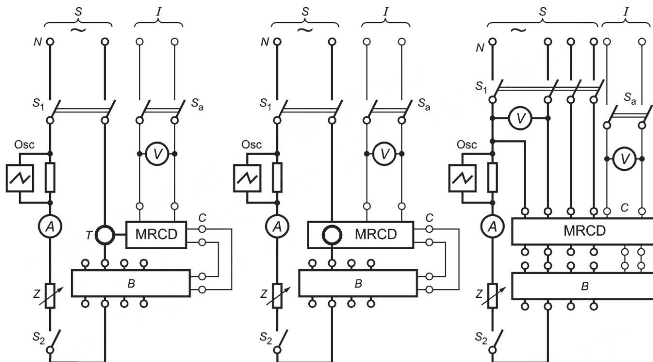
б) Модульное устройство защиты от тока утечки со встроенным сенсорным элементом
