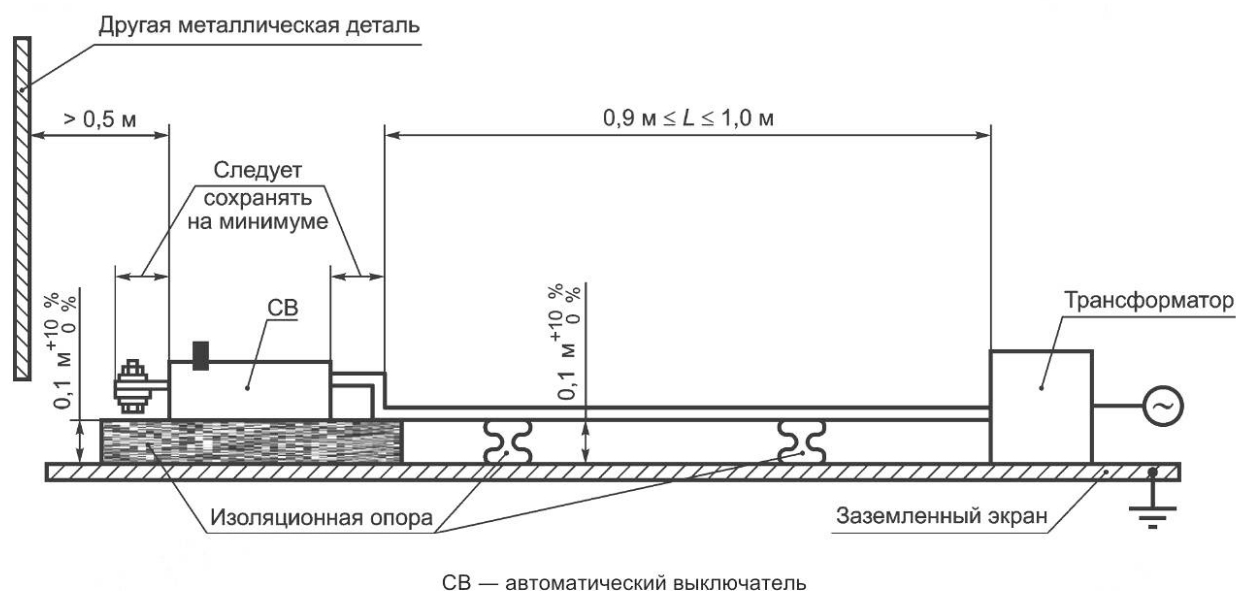
Рисунок F.20 — Общая схема испытания для проверки устойчивости к кондуктивным помехам, создаваемым полями высокой частоты (помехи общего вида)
