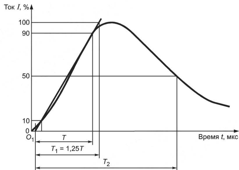
Рисунок В.6 — Волна импульсного тока 8/20 мкс
