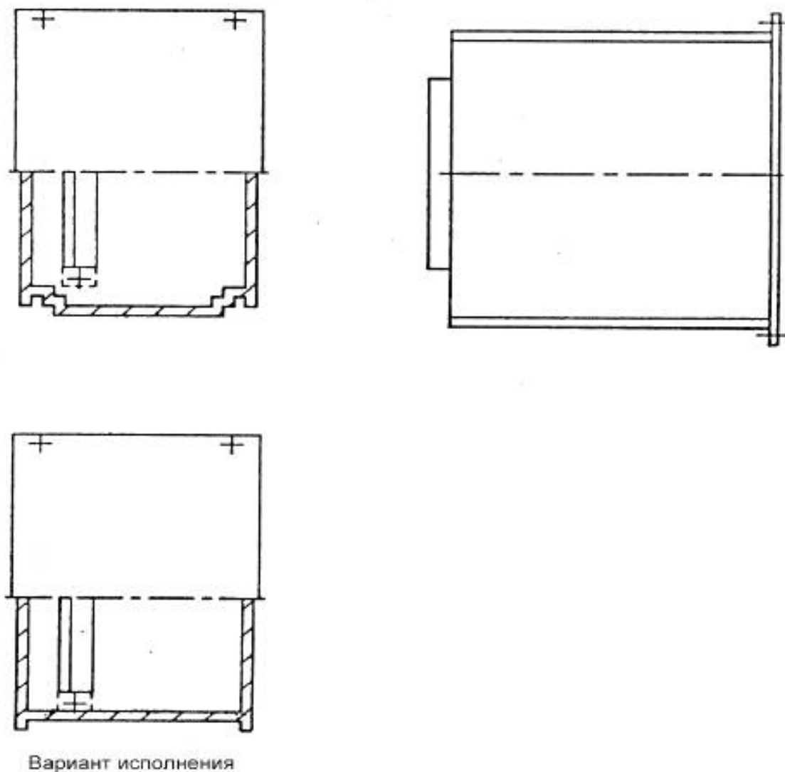
Рисунок 18 – Вставные частичные каркасы типа М
