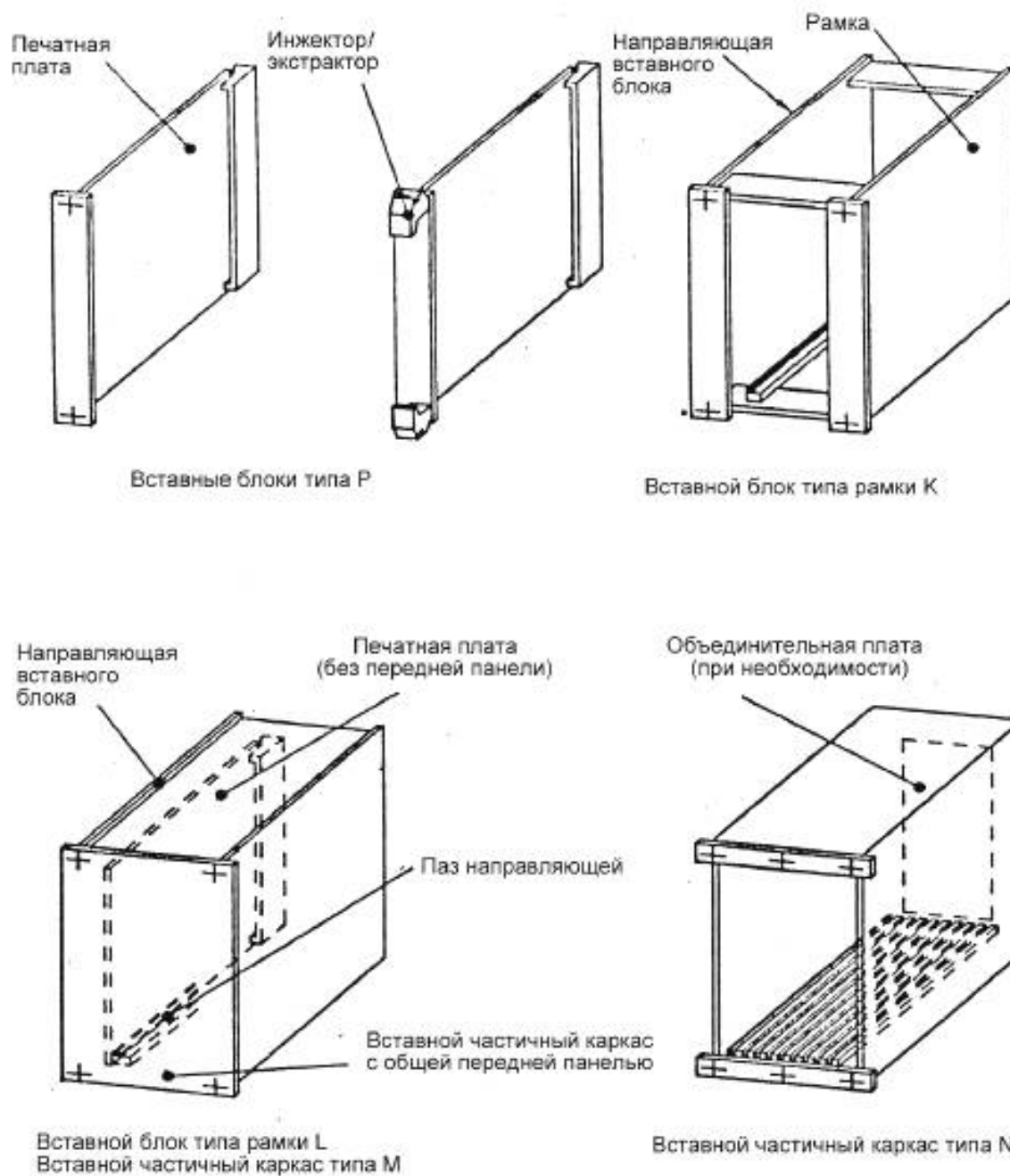
Рисунок 11 – Примеры типов вставных блоков
