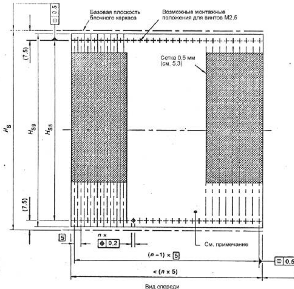
Рисунок 7 – Размеры объединительной платы
