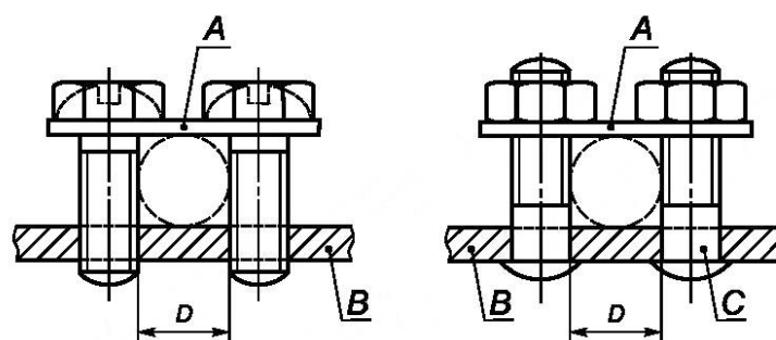
A — планка; B — неподвижная часть; C — штырь; D — канал для проводника
