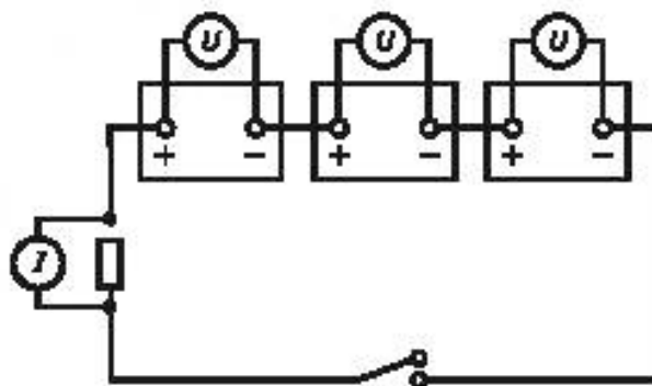
Рисунок 2 — Типичная электрическая схема при испытаниях
