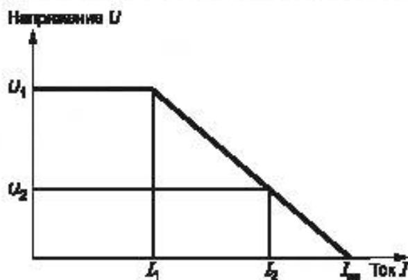
Рисунок 1 — Разрядная характеристика U = f(I)
