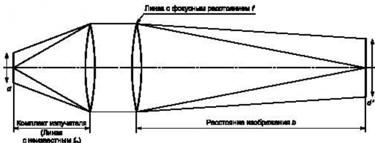
Рисунок 10 — Определение углового размера источника
