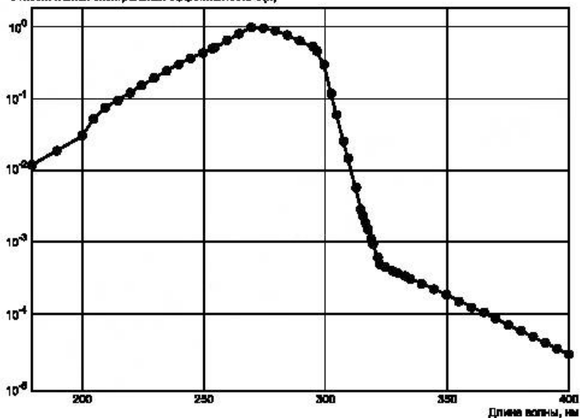
Относительная спектральная эффективность S(\lambda)
