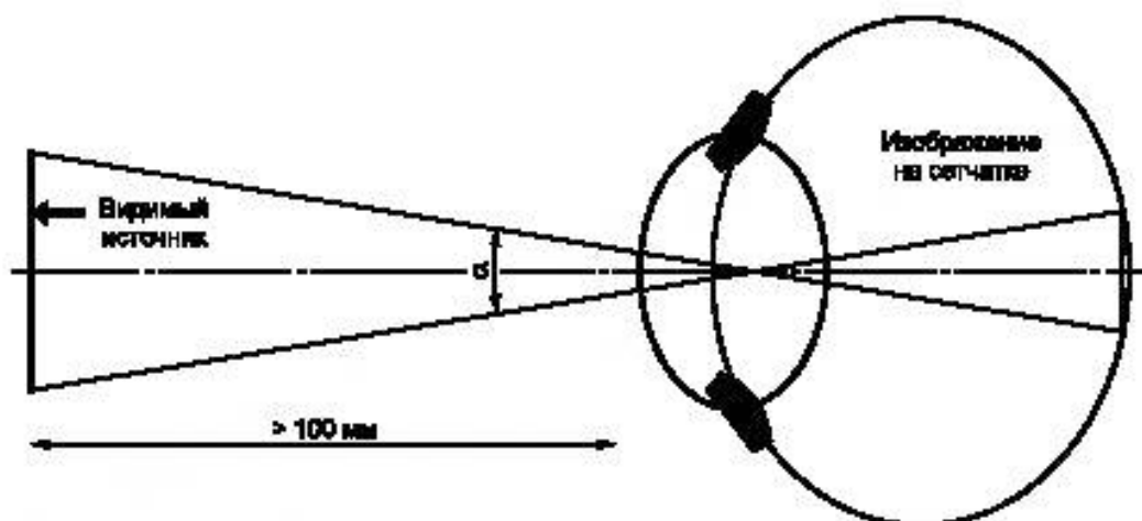
Рисунок 1 — Определение углового размера «видимого источника»
