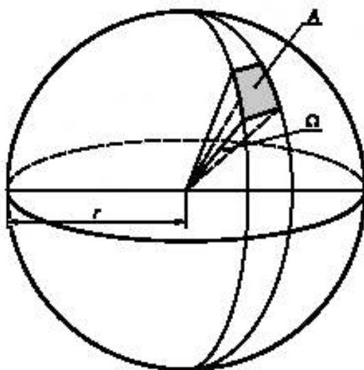
Рисунок 3 — Определение телесного угла
