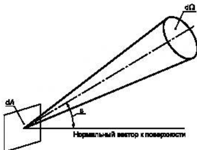
Рисунок 2 — Определение энергетической яркости
