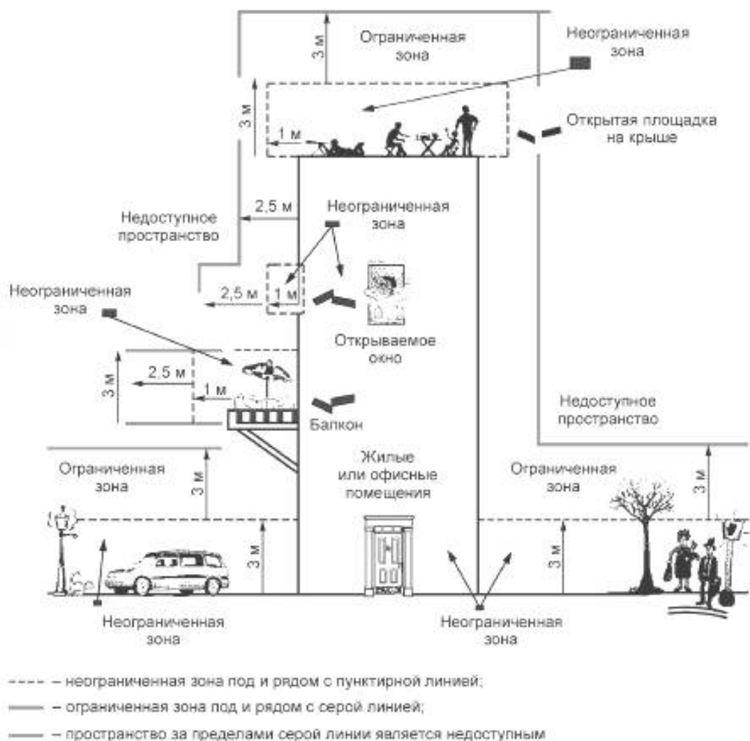
Рисунок 3 — Примеры вариантов внешнего расположения
