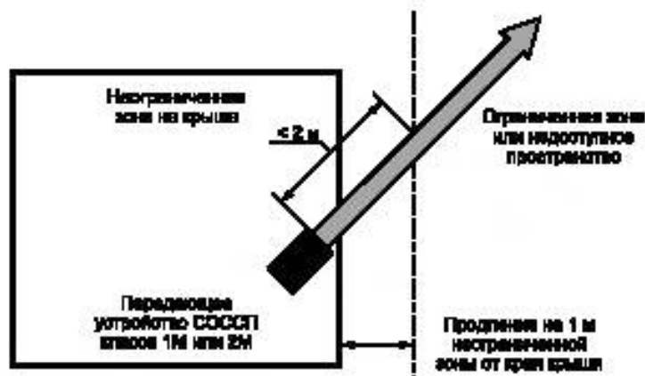
Рисунок 4 — Передаточное устройство лазеров класса 1М или 2М вблизи края крыши в неограниченной зоне
