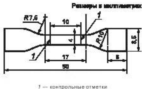
Рисунок 2 — Образец в виде двусторонней лопатки уменьшенного размера
