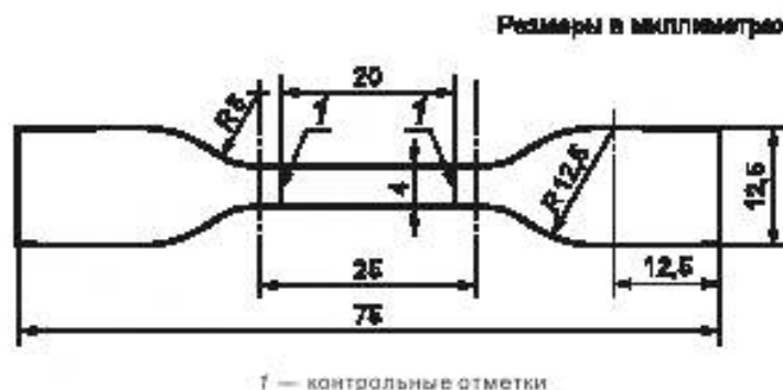
Рисунок 1 — Образец в виде двусторонней лопатки
