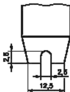
Рисунок 14 — Конец вырубного ножа с выемкой
