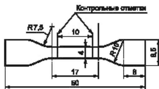
Рисунок 13 — Образец в виде лопатки уменьшенного размера
