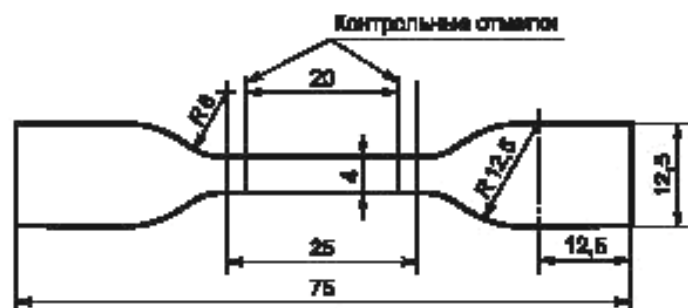
Рисунок 12 — Образец в виде двусторонней лопатки
