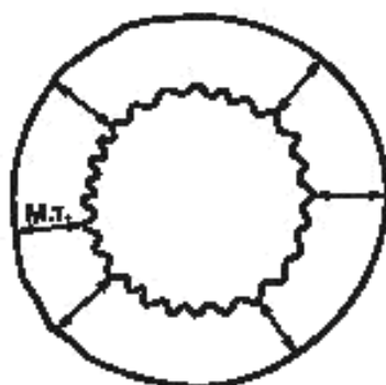
Рисунок 3 — Измерение толщины изоляции (многопроволочная жила)
