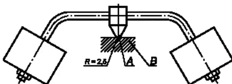
Рисунок 5 — Испытательное устройство для вдавливания шарика
