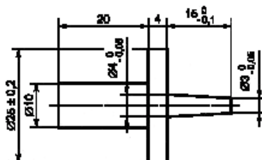
Рисунок 2 — Испытательный щуп
