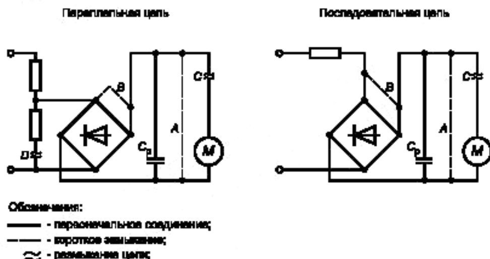
Рисунок В.1 — Схема имитации неисправностей
