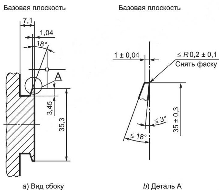
Рисунок 2 — Т-образная монтажная рейка ТН 35
