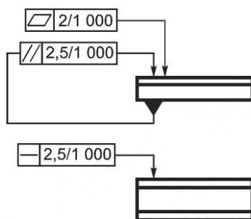
Рисунок A.2 — Допуски (ТН 15-5,5)
