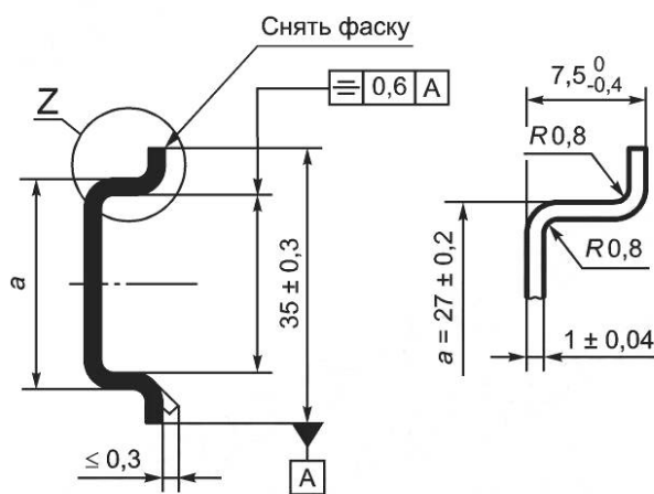
Деталь Z
