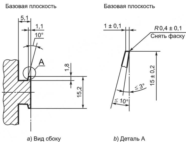
Рисунок 1 — Т-образная монтажная рейка ТН 15
