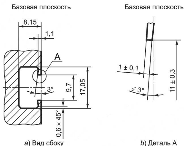
Рисунок 4 — С-образная монтажная рейка С 20
