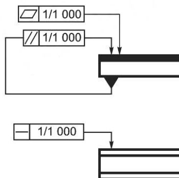
Рисунок A.4 — Допуски (ТН 35-7,5 и ТН 35-15)
