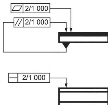
Рисунок A.4 — Допуски (ТН 35-7,5 и ТН 35-15)
