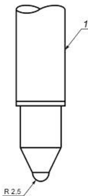
1 — нагрузочный шток
