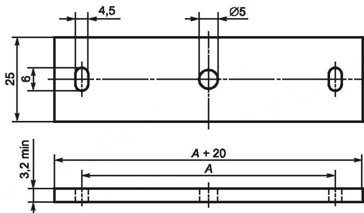
Рисунок 25 — Жесткая вставка
