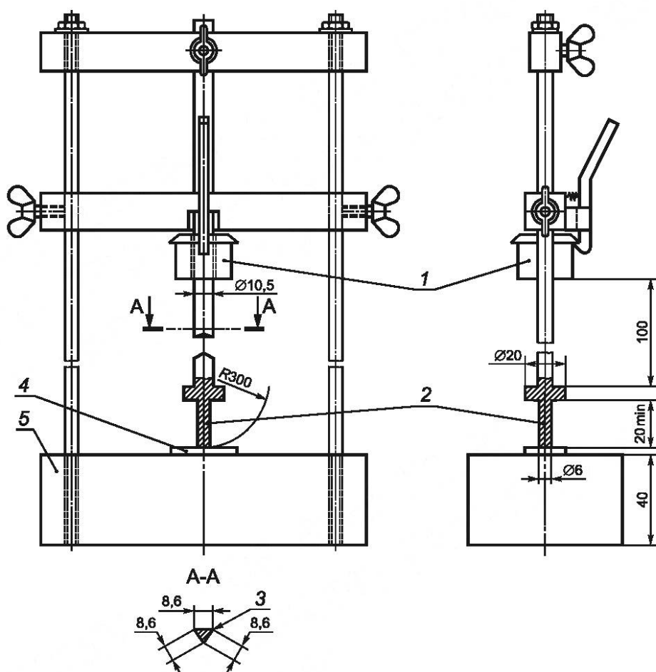
Рисунок 21 — Установка для испытаний на удар при низкой температуре
