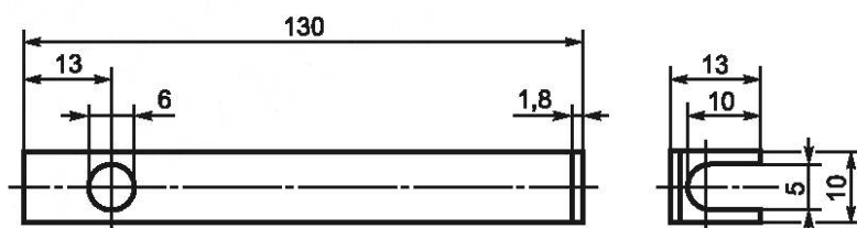
Рисунок 4 — Испытательная жила
