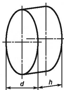
Рисунок 18б) — Контрольные площади поверхности круглых коробок и корпусов
