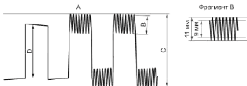
Рисунок 107 – Схема цепи для проверки линейности (см. 51.107.2)
