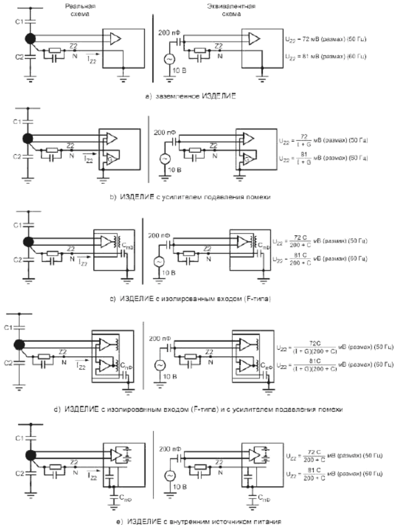
Рисунок FF.2 – Типичные схемы входных цепей ЭЛЕКТРОКАРДИОГРАФА и их эквивалентные схемы
