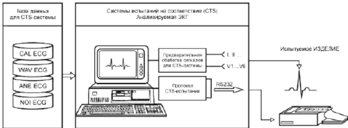
Рисунок II.1 – Система испытаний изделия на соответствие (CTS-система)
