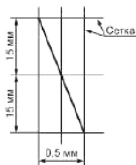
Рисунок 109 – Проверка прямоугольности системы координат (см. 51.108.4.1)
