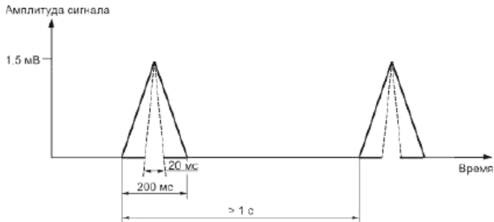
Рисунок 105 – Импульсы треугольной формы для испытания типа E (см. таблицу 114 и 51.107.1.1.1)
