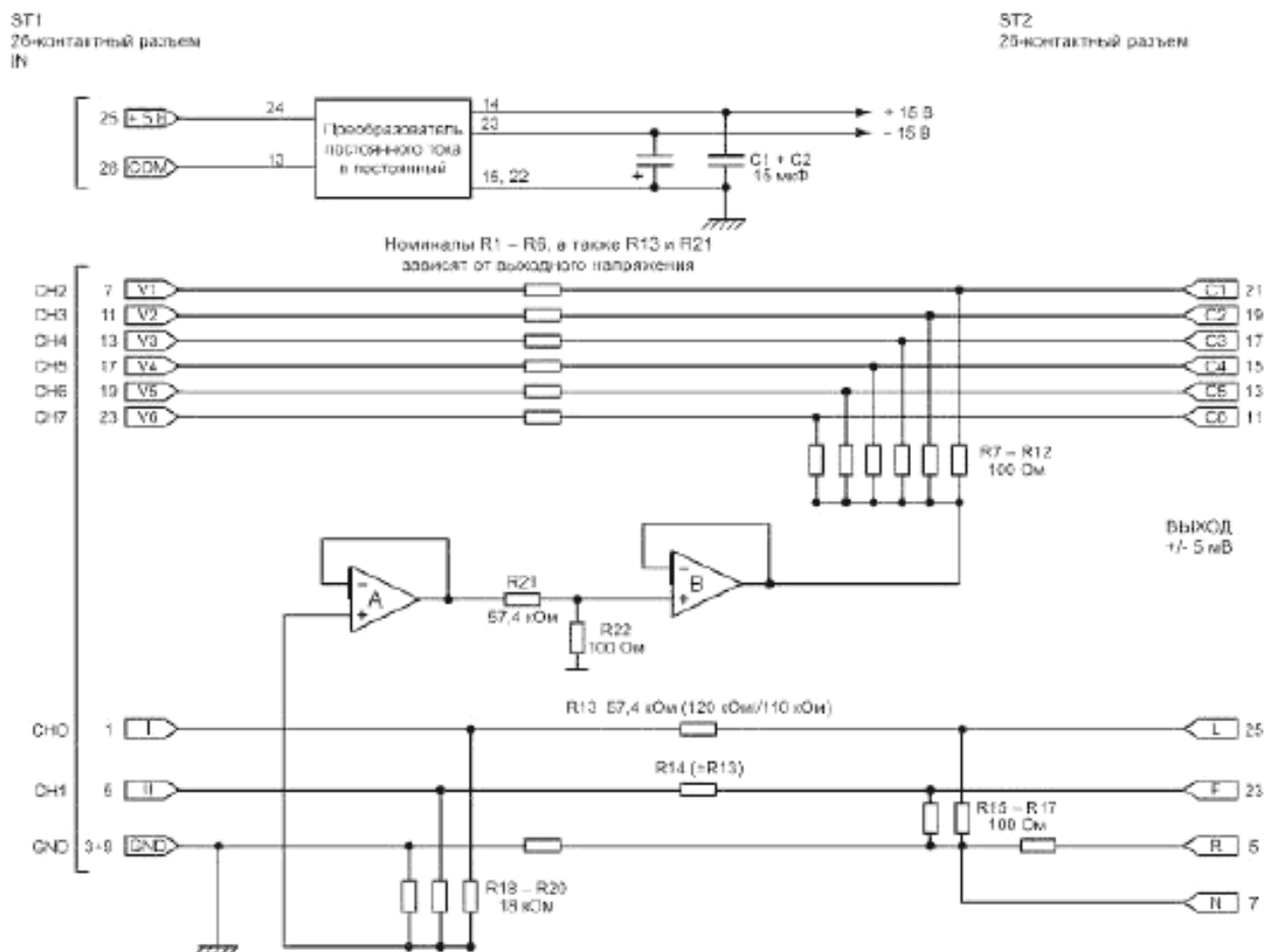
Рисунок II.2 – Пример схемы предварительной обработки ЭКГ-сигналов
