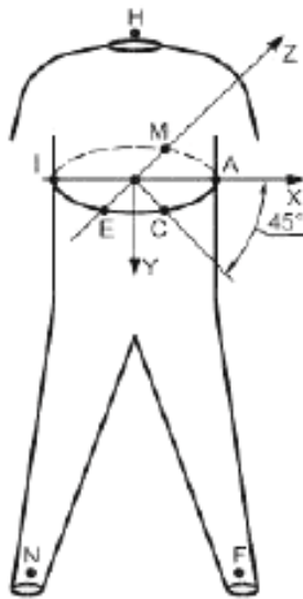
Рисунок 101 – Расположение электродов по методу Франка (см. таблицу 101)
