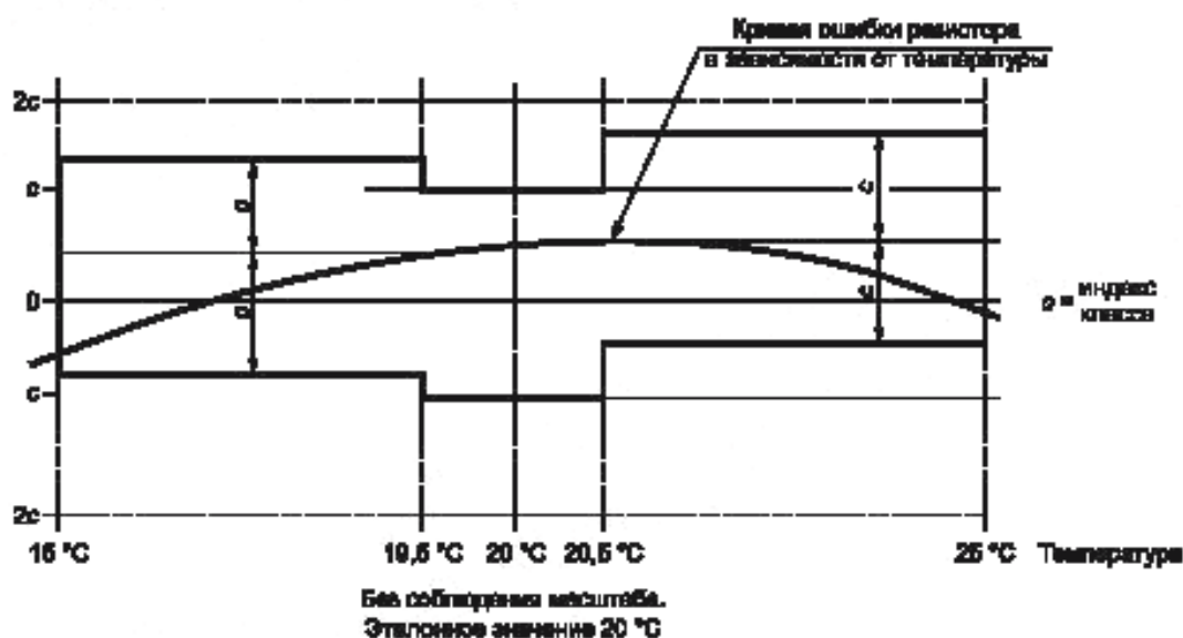
Рисунок 1 — Влияние температуры
