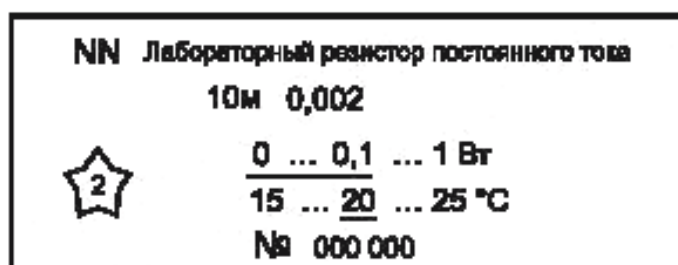
Рисунок 2 — Пример маркировки единичного резистора
