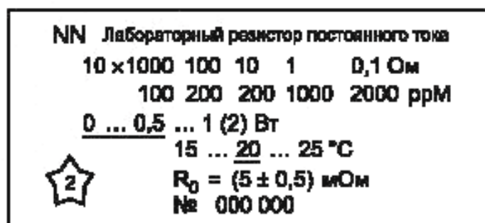
Рисунок 3 — Пример маркировки пятидекадного резистора
