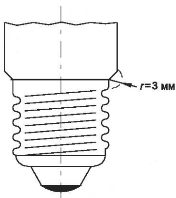
Рисунок 1 — Цоколь с резьбой Эдисона
