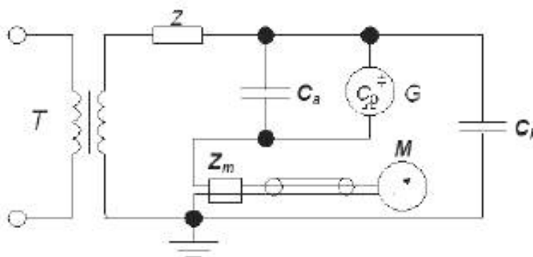
Рисунок В.3 – Пример симметричной испытательной схемы
