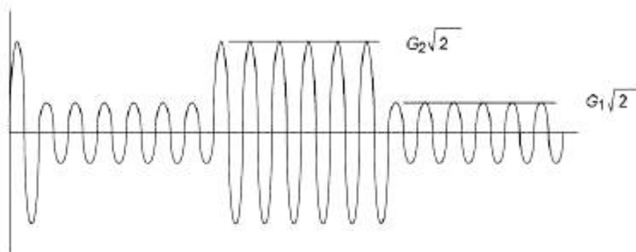
Рисунок 12 — Испытательная осциллограмма
