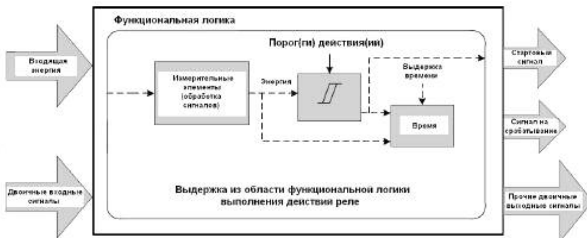
Рисунок 1 — Функциональный блок диаграмм выполнения защиты
