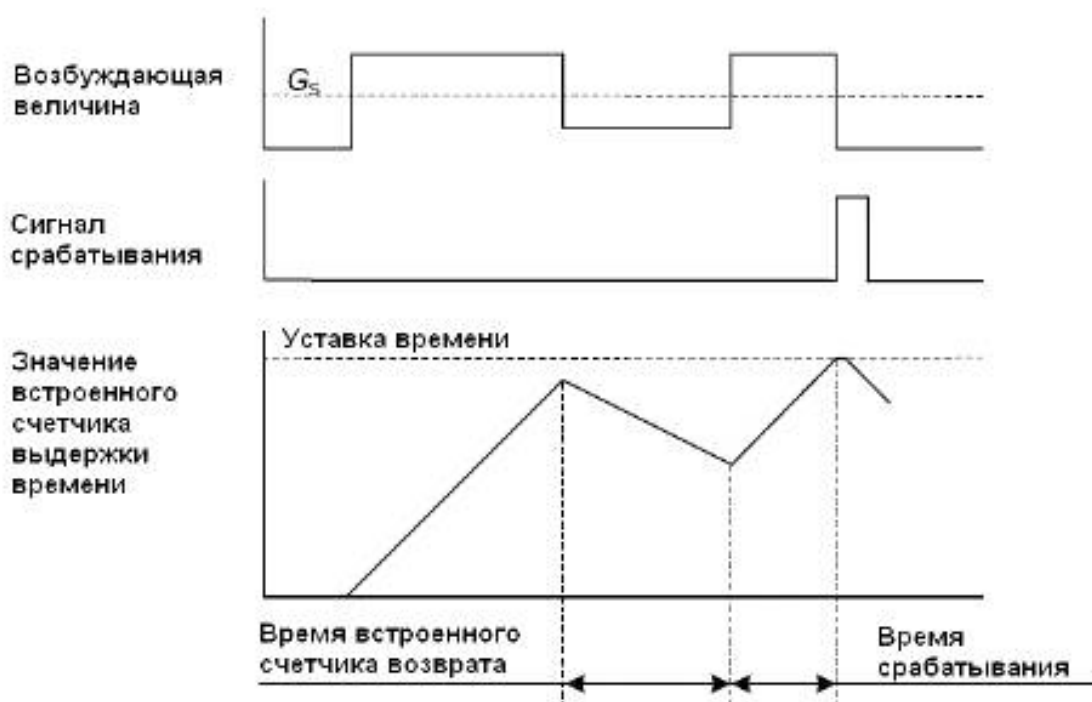
Рисунок А.1 — Определение зависимости времени возврата
