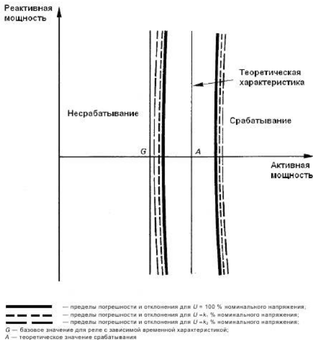
Рисунок 1 — Характеристика срабатывания реле мощности
