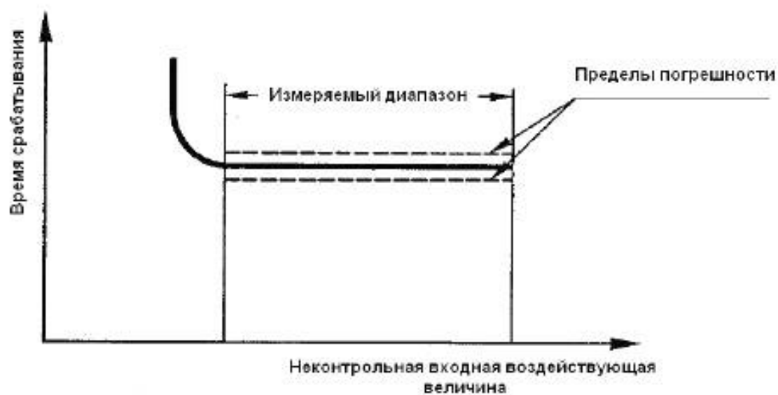
Рисунок 6 — Время срабатывания для реле мощности с независимой временной характеристикой
