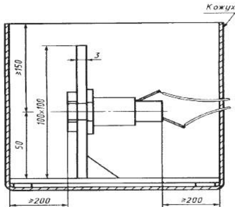
Рисунок 9 — Испытательное устройство
