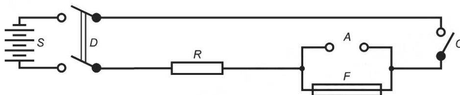
Рисунок А.1 б) — Типовая испытательная схема для испытаний отключающей способности плавких вставок с отключающей способностью менее или равной 100 А
