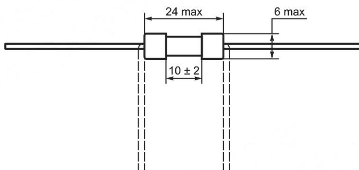
Рисунок А.2 — Испытательное основание
