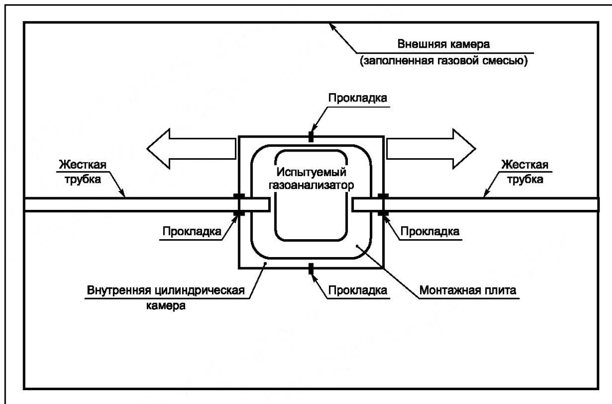
Рисунок В.2 — Пример применения испытательной камеры (вариант 1)
