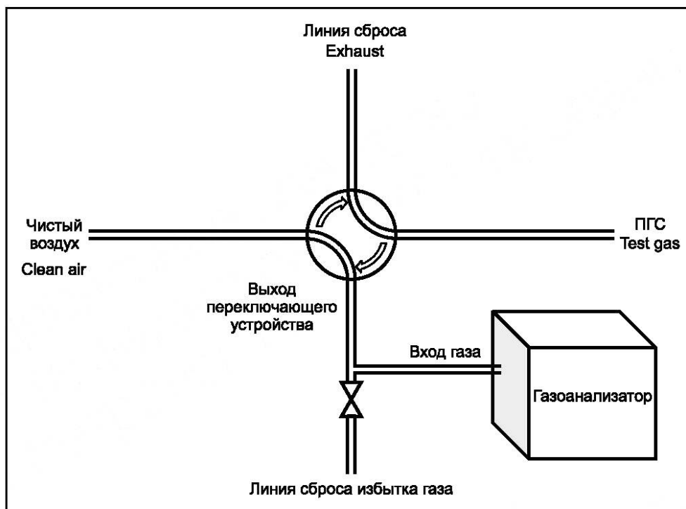
Рисунок В.1 — Схематическое изображение испытательной установки
