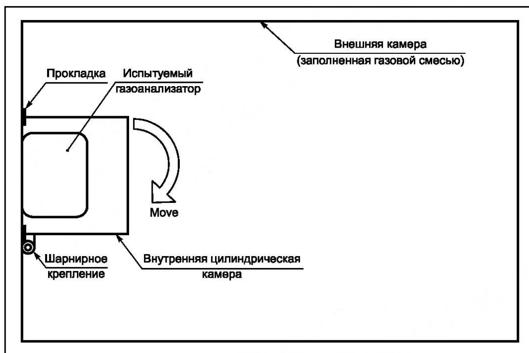
Рисунок В.4 — Пример применения испытательной камеры (вариант 5)
