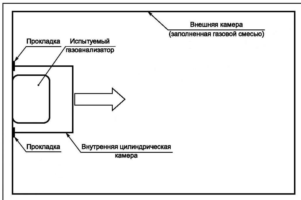
Рисунок В.3 — Пример применения испытательной камеры (вариант 2)
