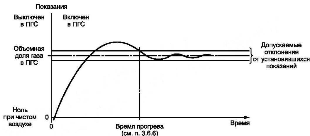
Рисунок 2 — Время прогрева в ПГС
