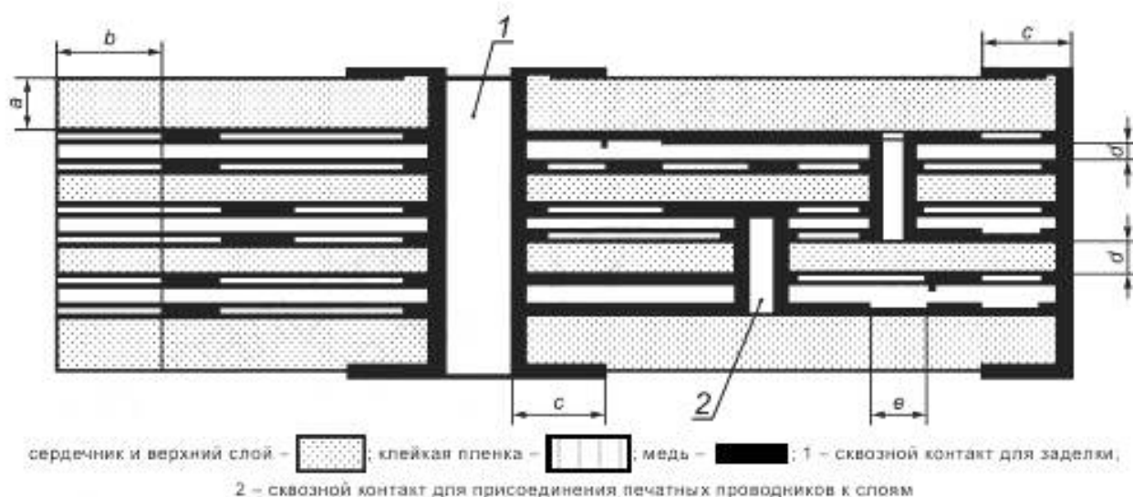
Рисунок 2 – Минимальные расстояния для многослойных печатных монтажных плат.
