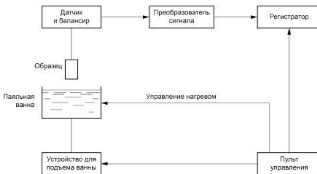
Рисунок 1 — Блок-схема для испытания
