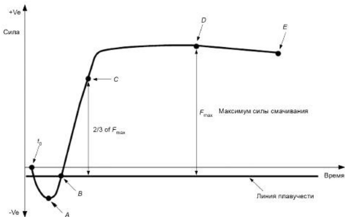
Рисунок 2 — Условия смачивания
