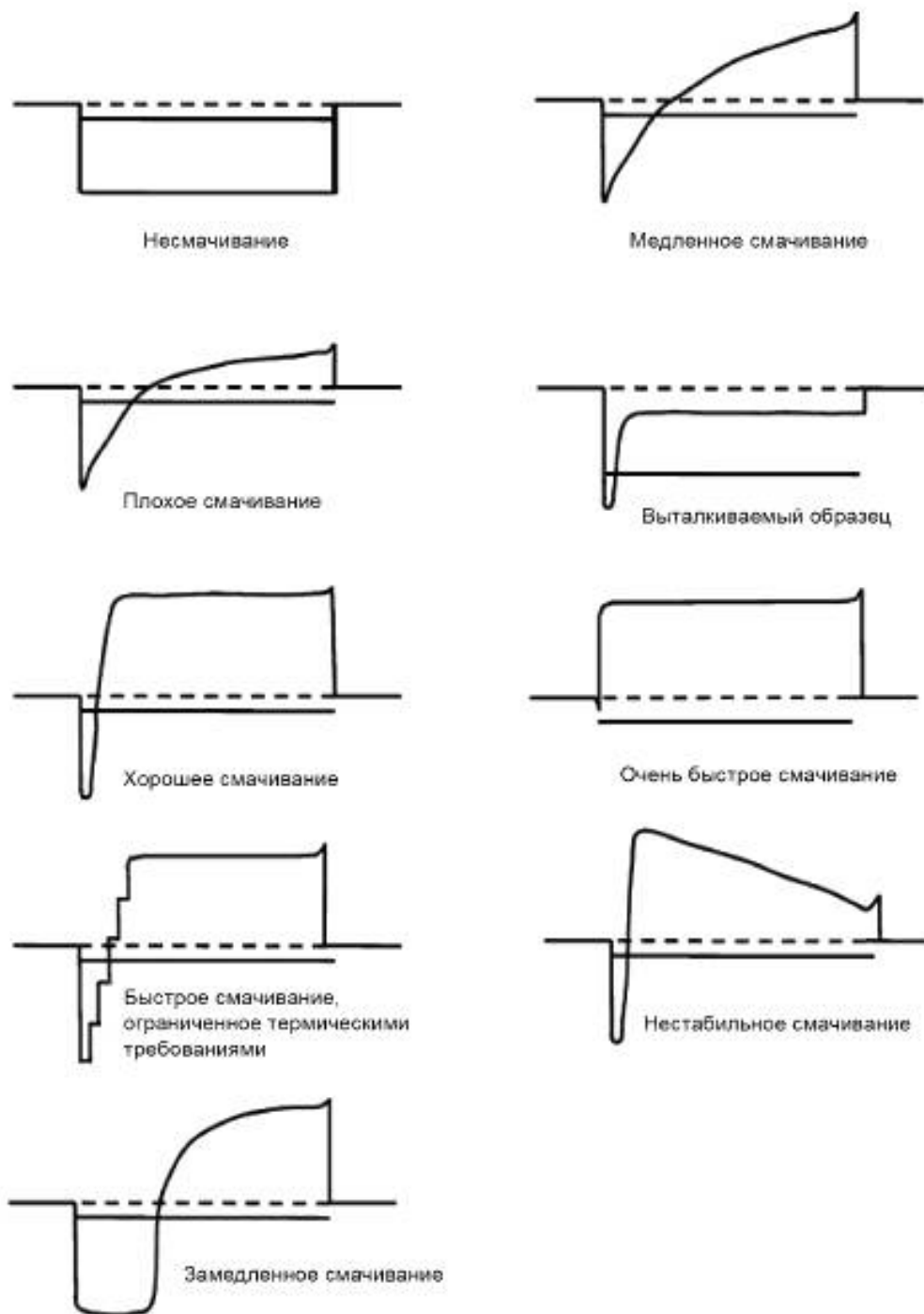
Рисунок В.1 — Характерные кривые «сила — время»
