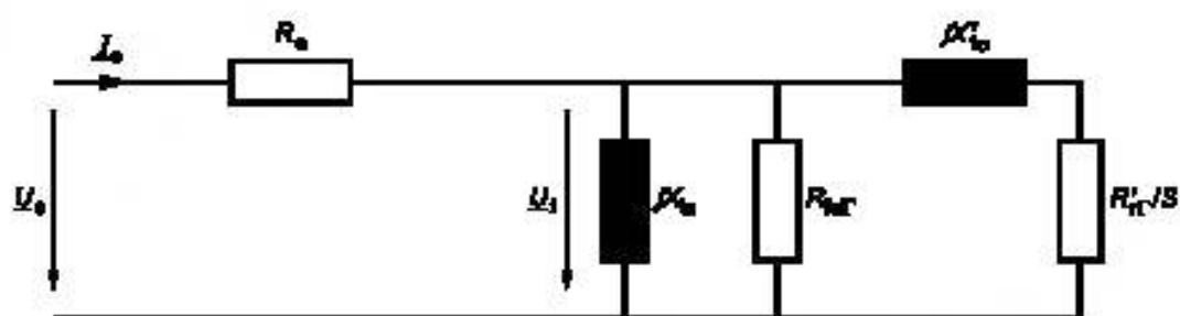
Рисунок 4 — Г-образная схема замещения
