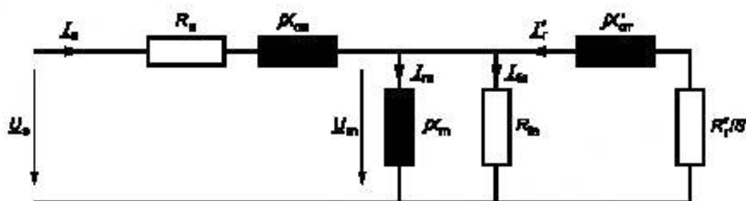
Рисунок 1 — Т-образная схема замещения
