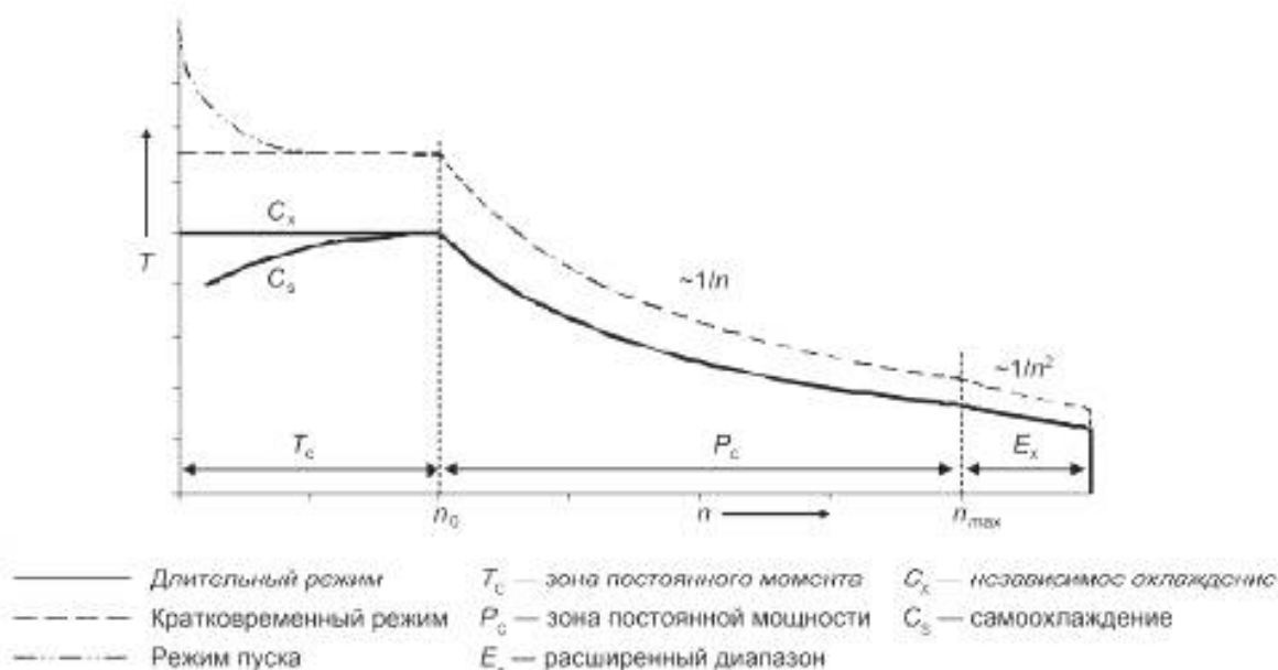
Рисунок 1 — Допустимая область формирования механических характеристик
