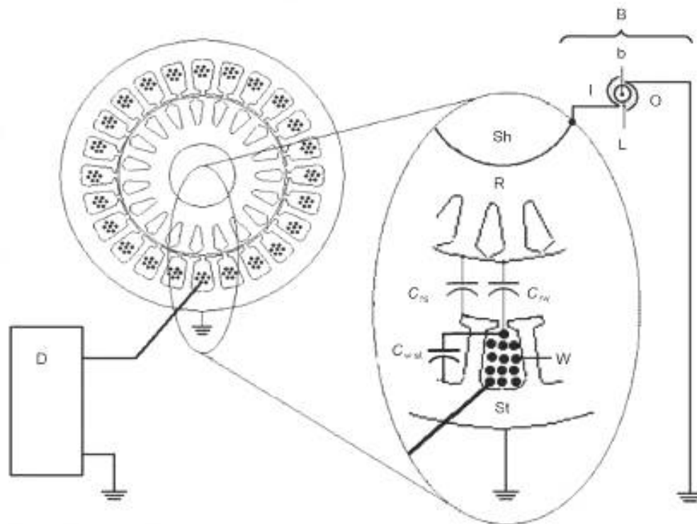
D — преобразователь; Sh — вал; R — ротор; St — статор; W — обмотка; C_{rs} — емкость ротор-статор; C_{rw} — емкость обмотки ротора; C_{ws} — емкость обмотки статора; B — подшипник; b — шарики или ролики; I — внутреннее кольцо; O — внешнее кольцо; L — пленка смазки
