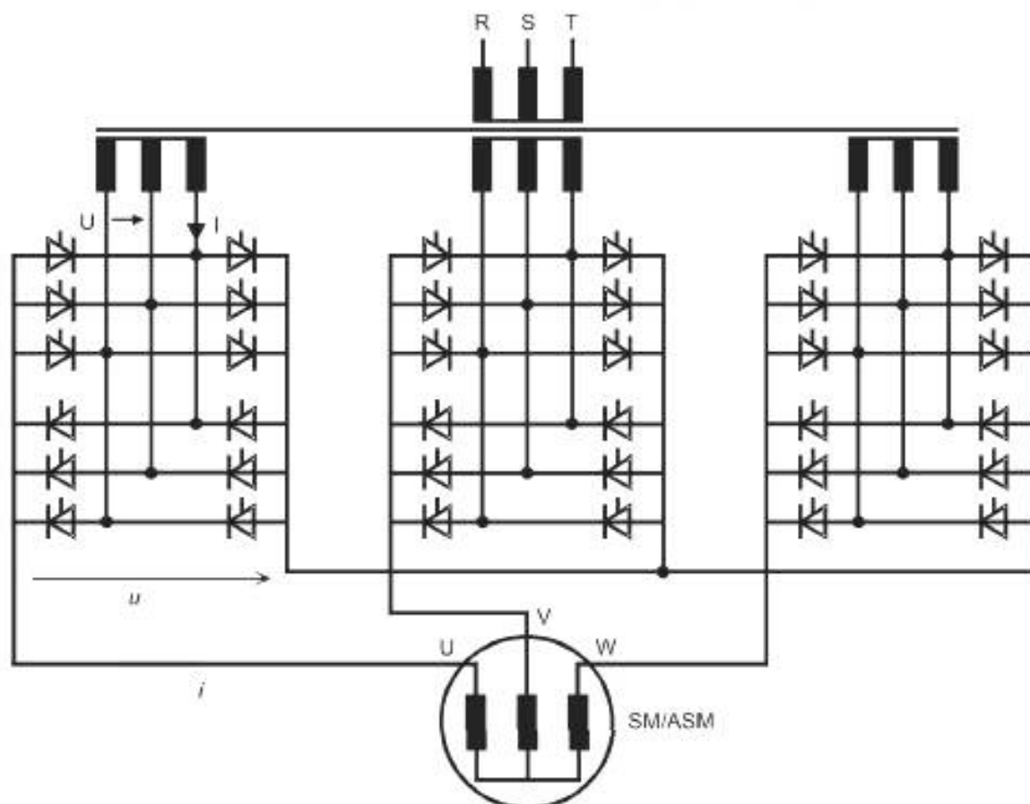
Рисунок 36 — Схема циклоконвертора
