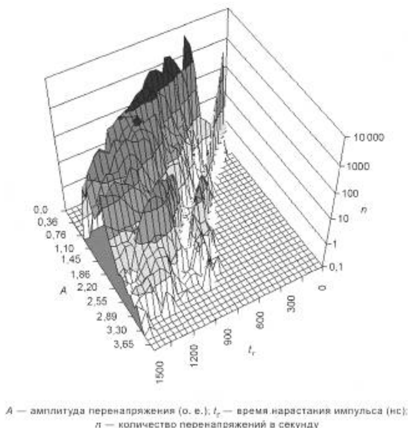
Рисунок 9 — Диаграмма перенапряжений на клеммах двигателя при питании от ШИМ-преобразователя
