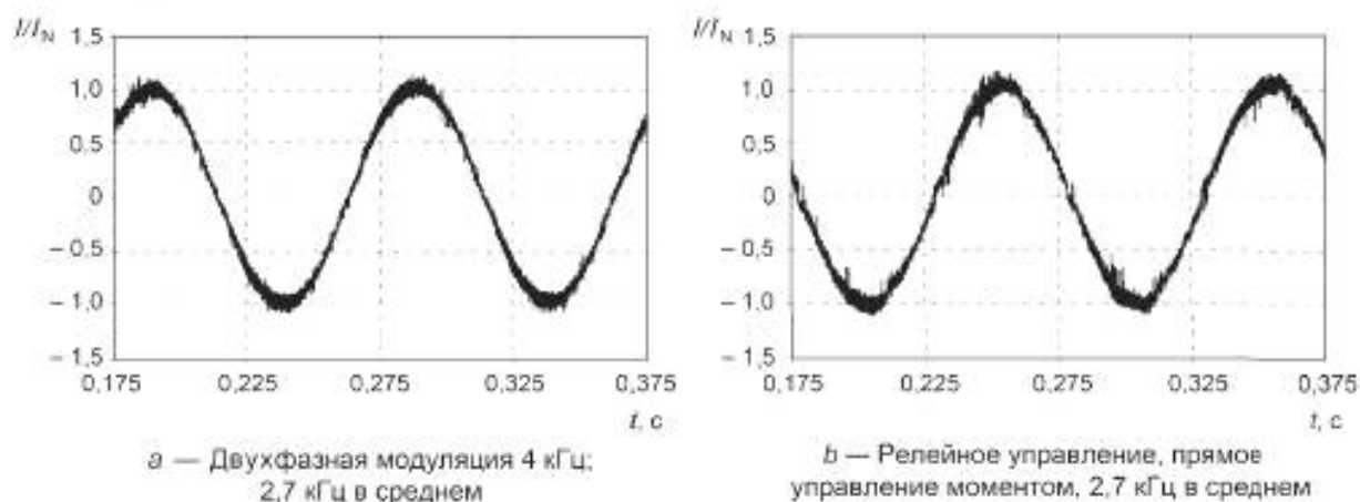
Рисунок В.6 — Типичные осциллограммы тока машины
