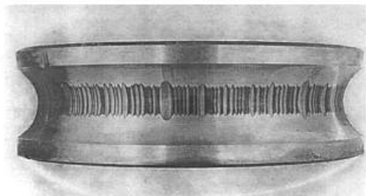
Рисунок 18 — Появление бороздок из-за чрезмерного тока в подшипниках
