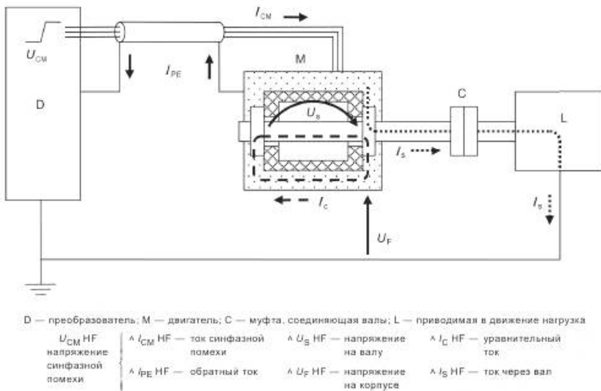
Рисунок 15 — Возможные токи, протекающие через подшипники
