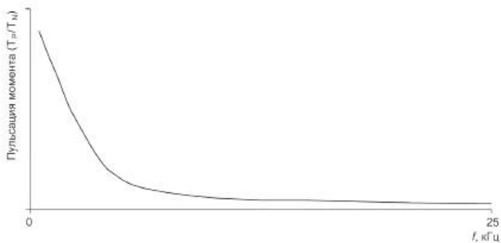
Рисунок А.3 — Влияние частоты коммутации на пульсации крутящего момента
