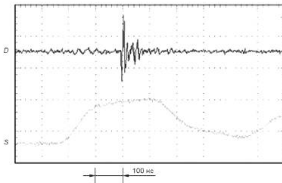
Рисунок 14 — Импульс разряда на клеммах двигателя (100 нс/деление)
