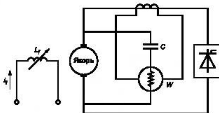
Рисунок 9 — Схема для измерения потерь от пульсирующих токов
