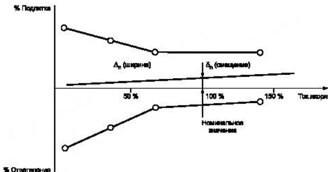
Рисунок 6 — Зона безыскровой коммутации при постоянной скорости вращения
