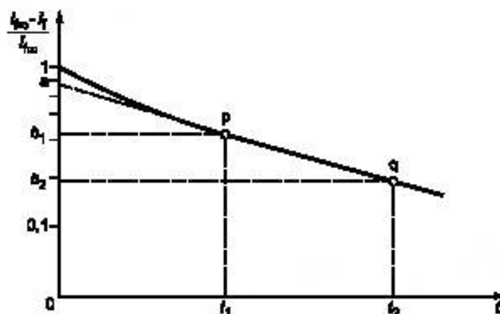
Рисунок 3 — Определение индуктивности обмотки возбуждения
