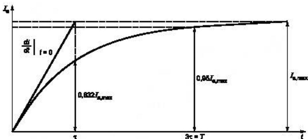
Рисунок 8 — Переходный процесс нарастания тока якоря
