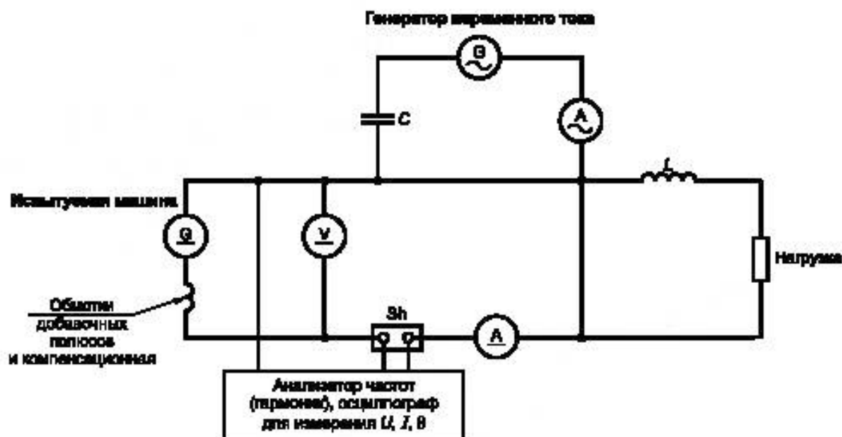
Рисунок 1 — Определение индуктивности цепи якоря с учетом насыщения
