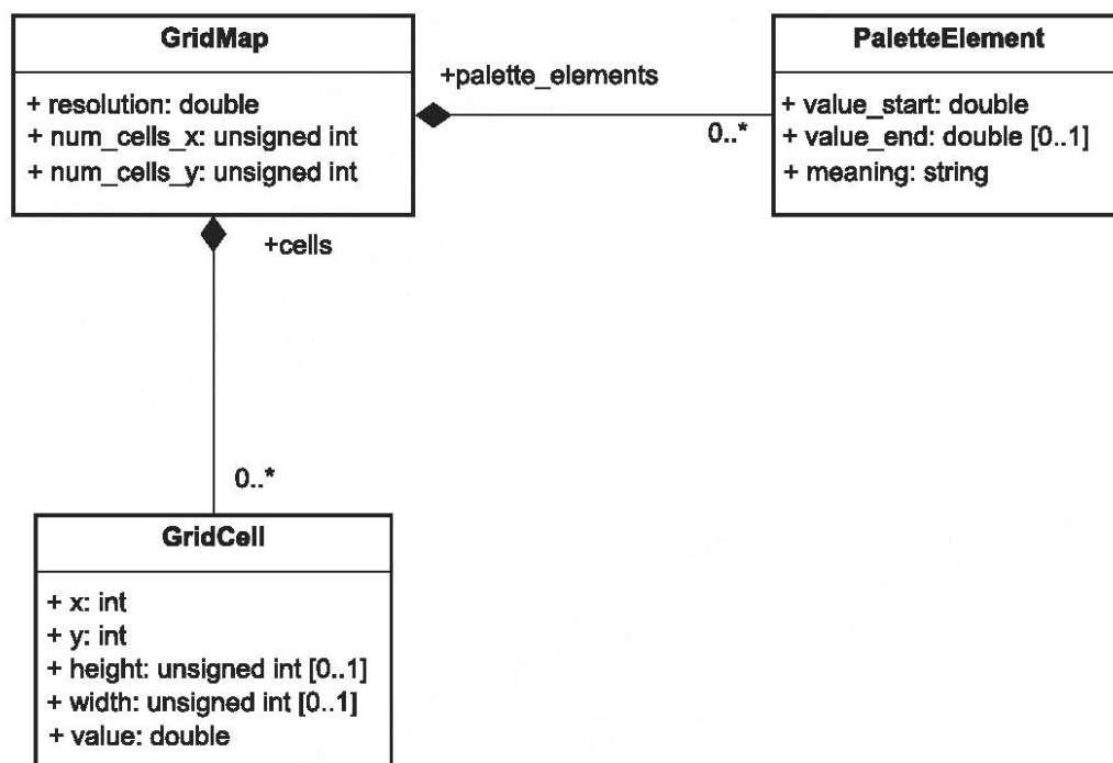
Рисунок 3 — UML-диаграмма карты с координатной сеткой
