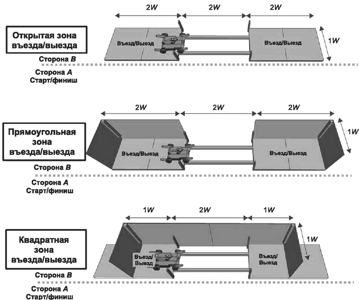
Рисунок 4 — Вид испытательного стенда с указанием размеров и обозначенными зонами въезда/выезда для открытой, ограниченной прямоугольной и ограниченной квадратной конфигураций
