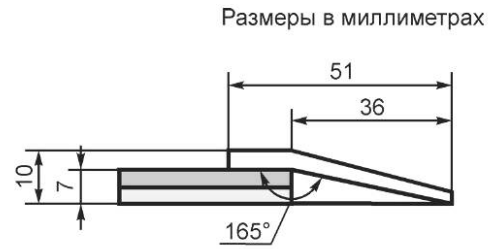
Рисунок А.2 — Иллюстрация установки металлической планки
