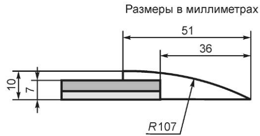
Рисунок А.3 — Иллюстрация установки деревянной планки
