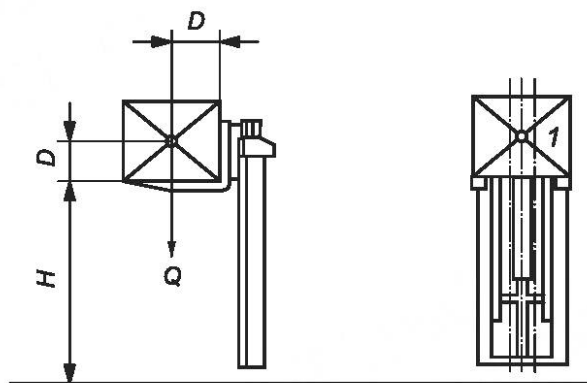
1 — центр массы груза, расположенный в продольной плоскости симметрии между вертикальными стойками грузоподъемного механизма; D — номинальное расстояние центра груза; H — номинальная высота подъема; Q — номинальная грузоподъемность
