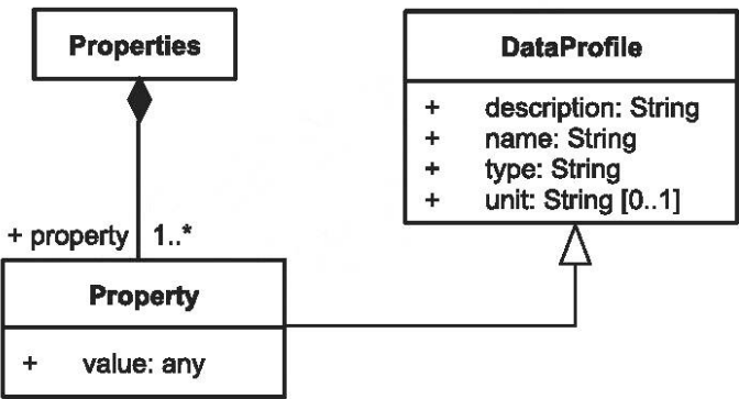
Рисунок 4.6 — Диаграмма классов для класса Properties
