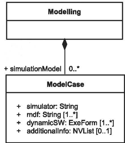
Рисунок 4.12 — Взаимосвязь между классами для класса Modelling
