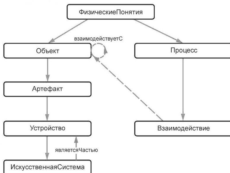
Рисунок 4 — Таксономия понятий ИскусственнаяСистема и Взаимодействие онтологии CORAX
