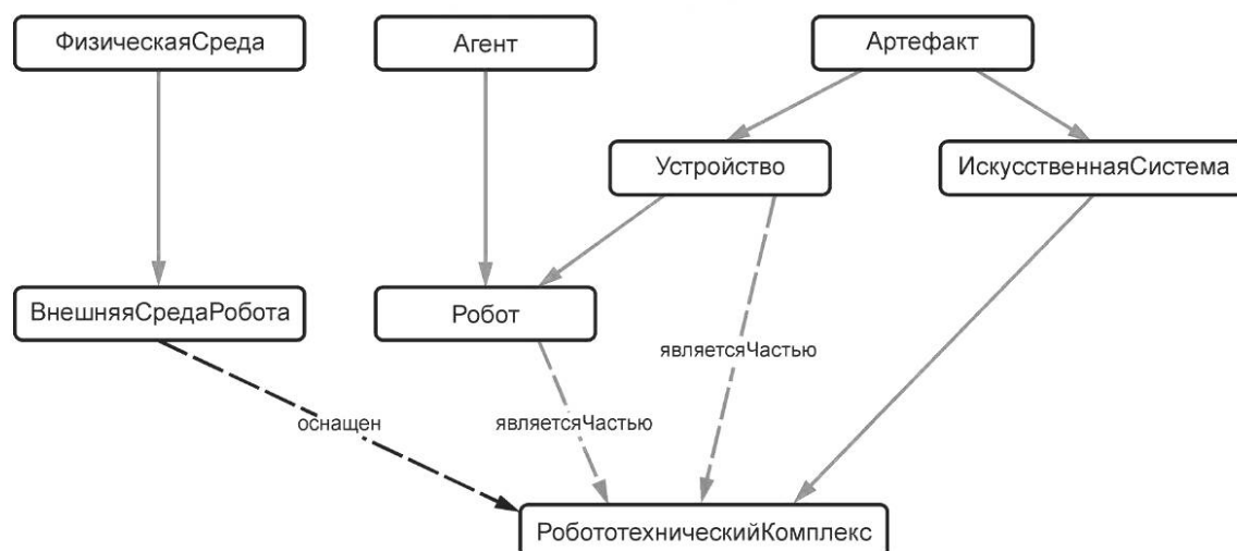
Рисунок 6 — Таксономия понятия РобототехническийКомплекс
