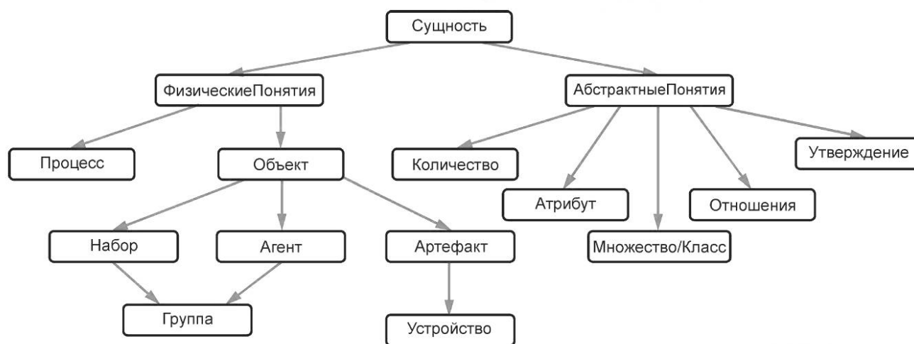
Рисунок 1 — Базовая таксономия SUMO
