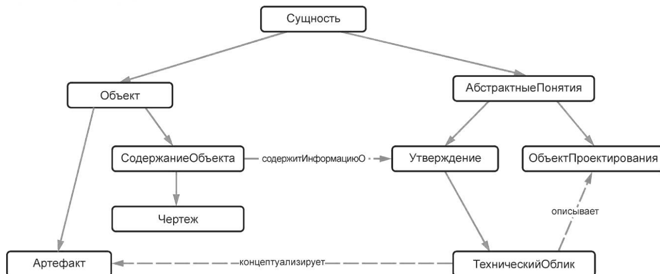
Рисунок 3 — Таксономия понятий ТехническийОблик и ОбъектПроектирования онтологии CORAX
