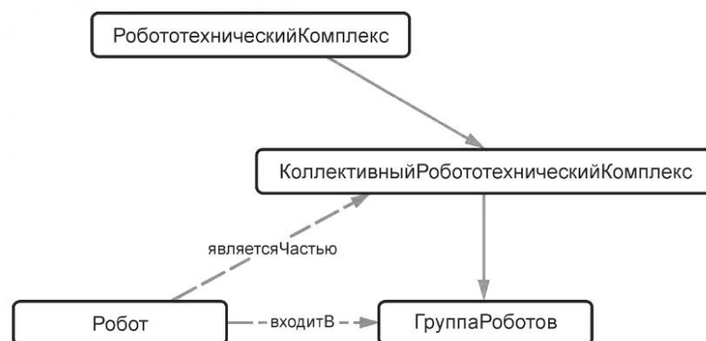
Рисунок 7 — Таксономия понятия КоллективныйРобототехническийКомплекс
