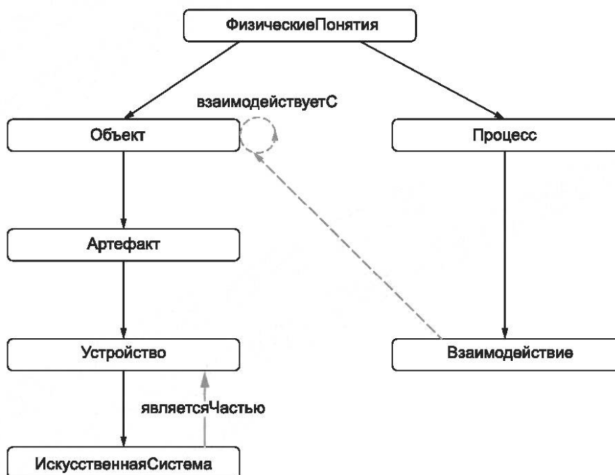
Рисунок 3 — Таксономия понятий ИскусственнаяСистема и Взаимодействие онтологии CORAX
