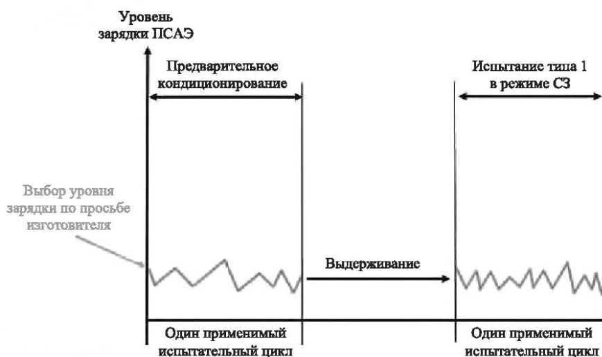
Рисунок Е.11 — ГЭМ-БЗУ и ГТСТЭ-БЗУ, испытание типа 1 в режиме сохранения заряда
