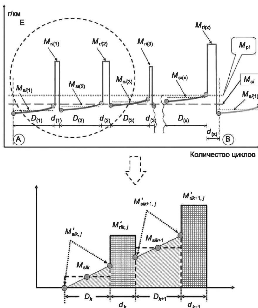
Рисунок Г.9 — Параметры, измеряемые в ходе испытания на выбросы во время циклов с регенерацией и между ними (условный пример)
