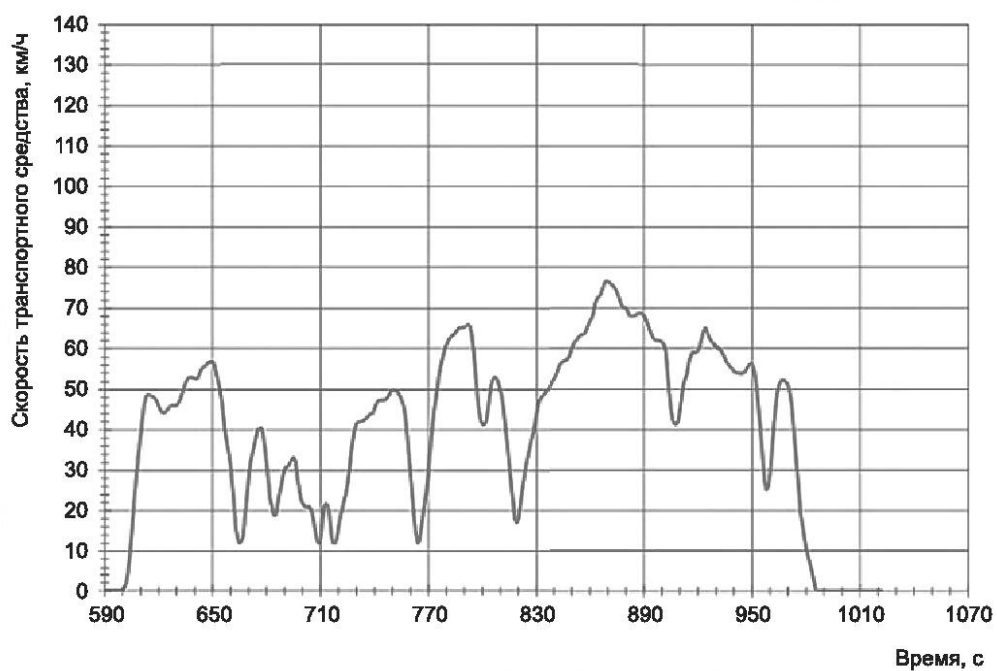
Рисунок А.9 — ВЦИМГ, цикл применительно к классу 3b, фаза Medium 3b
