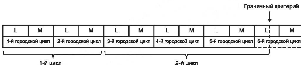
Рисунок Д.5 — Пример нечетного количества завершенных городских испытательных циклов, предшествующих городскому циклу, в ходе которого выполняется граничный критерий
