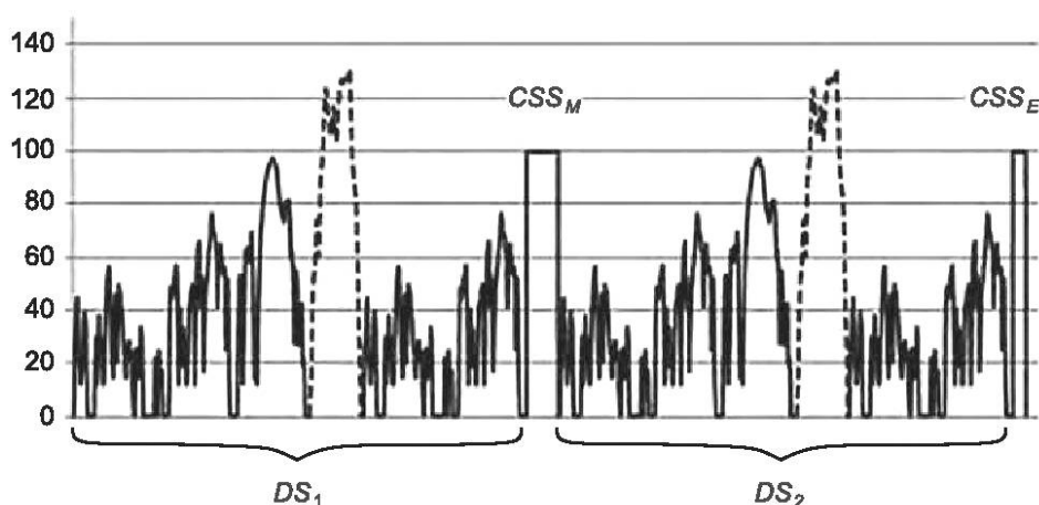
Рисунок Е.2 — Кривая скорости для сокращенной процедуры испытания типа 1
