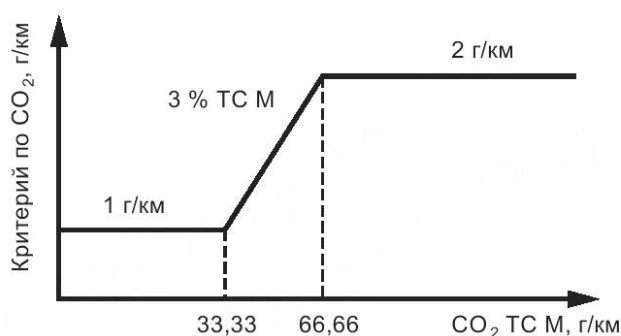
Рисунок Е.6 — Критерий линейности для ТС М
