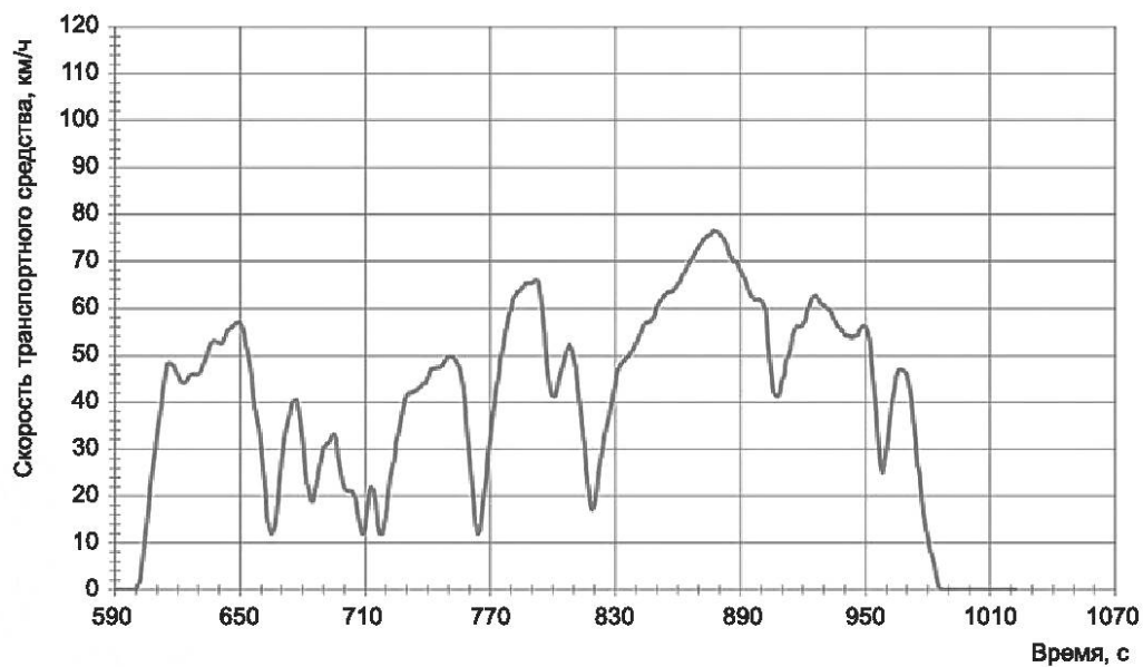
Рисунок А.8 — ВЦИМГ, цикл применительно к классу 3a, фаза Medium 3a
