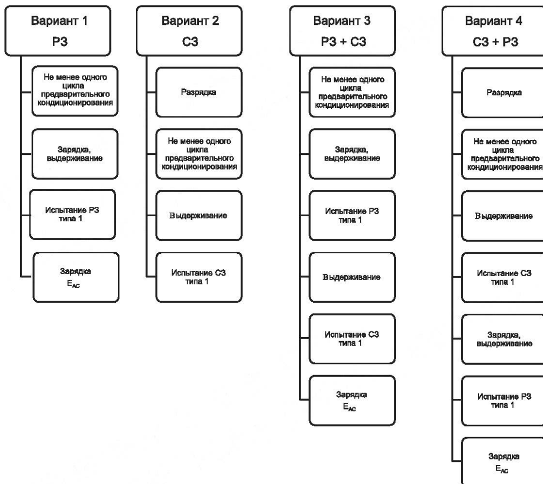
Рисунок Е.1 — Возможные варианты последовательности испытания ГЭМ-ВЗУ и ГТСТЭ-ВЗУ
