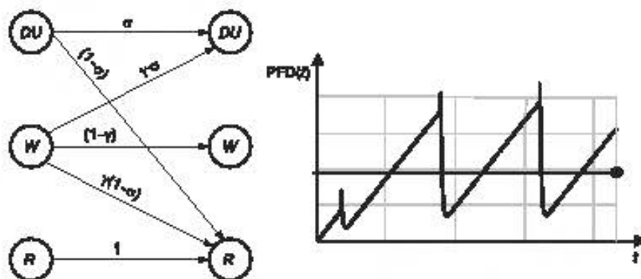
Рисунок Б.27 — Влияние на отказы самого запроса
