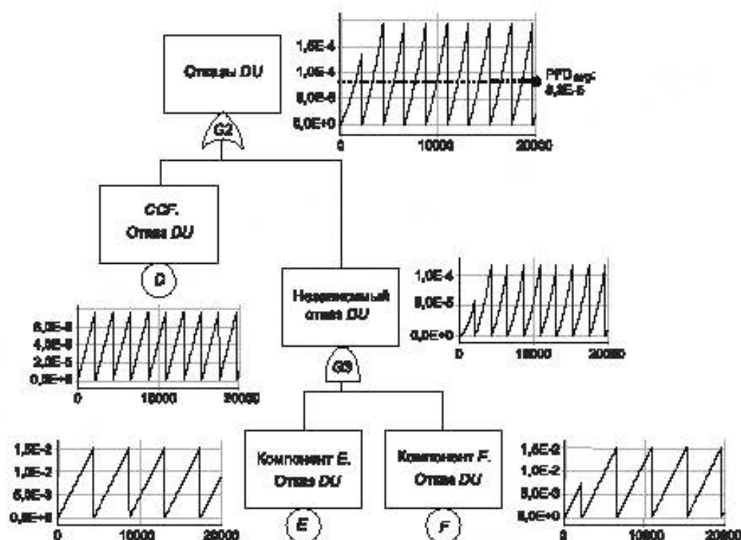
Рисунок Б.21 — Влияние смещения проверок
