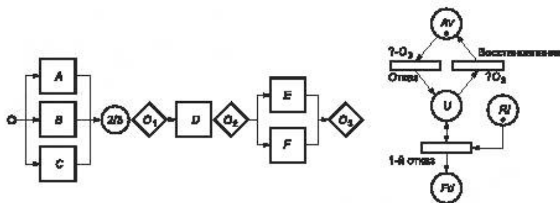
Рисунок Б.35 — Использование блок-схемы надежности для построения сети Петри и вспомогательной сети Петри для вычислений PFD и PFH
