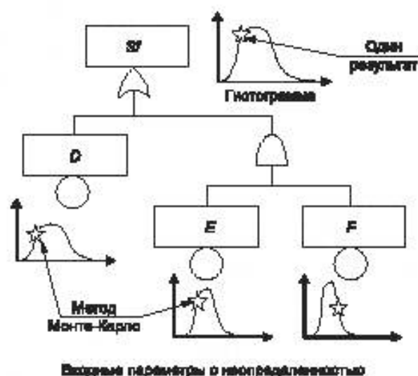
Рисунок Б.38 — Принцип распространения неопределенности
