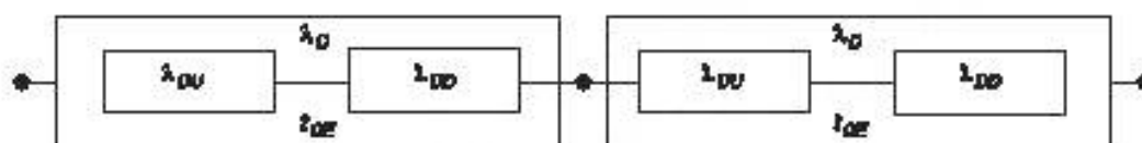
Рисунок Б.9 — Структурная схема надежности для архитектуры 2oo2
