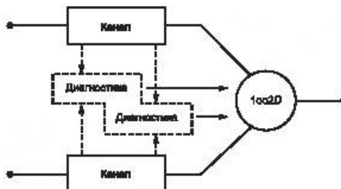
Рисунок Б.10 — Структурная схема архитектуры 1oo2D
