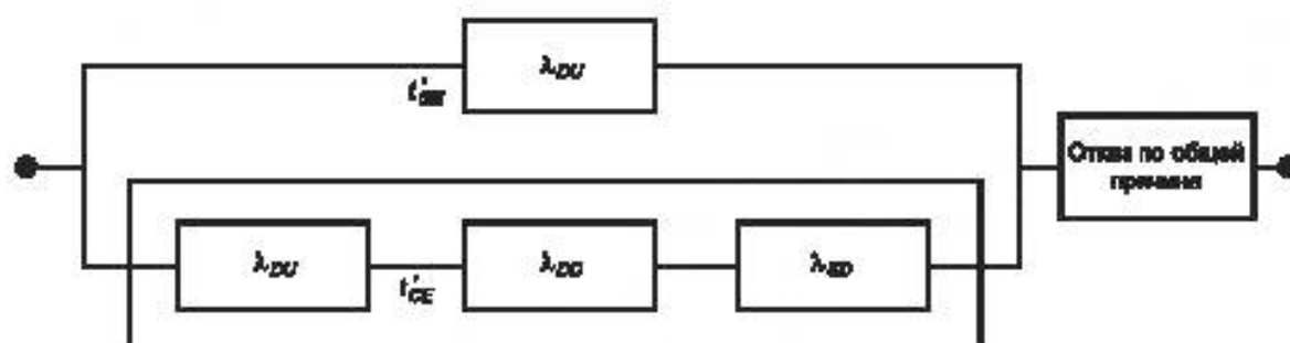
Рисунок Б.11 — Структурная схема надежности для архитектуры 1oo2D
