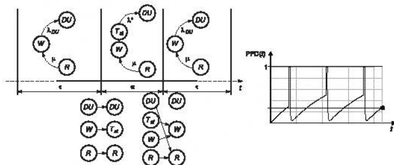
Рисунок Б.28 — Моделирование влияния продолжительности проверки
