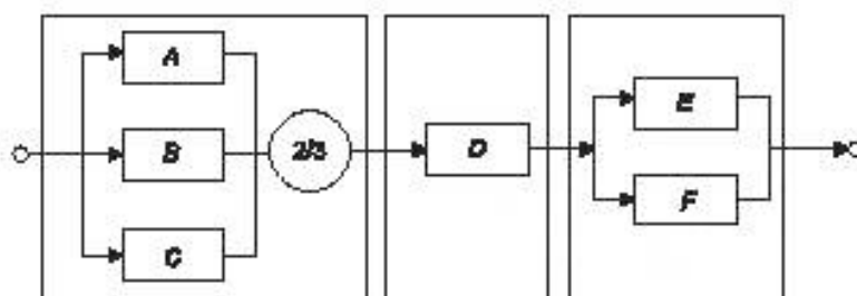
Рисунок Б.16 — Блок-схема надежности простой полной СБЗС системы с датчиками, организованными по схеме 2oo3
