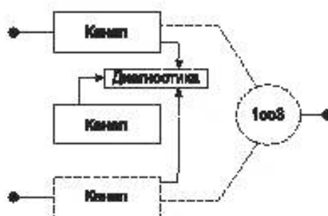
Рисунок Б.12 — Структурная схема архитектуры 2oo3
