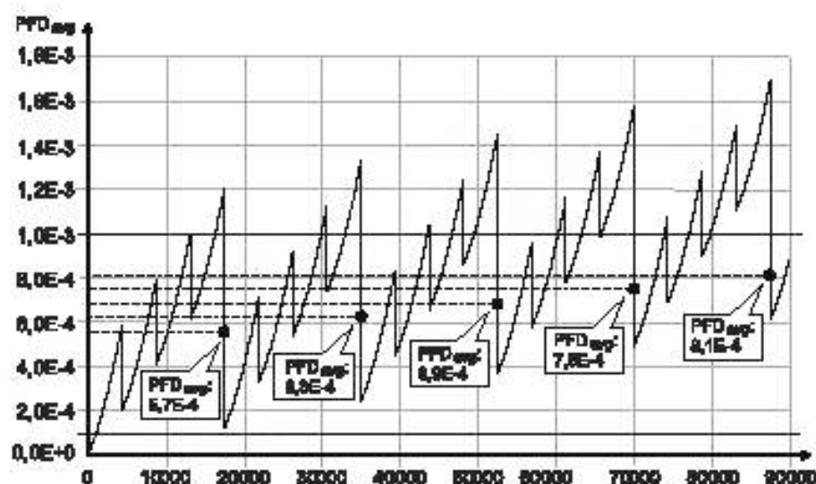
Рисунок Б.22 — Пример комплексного шаблона проверки
