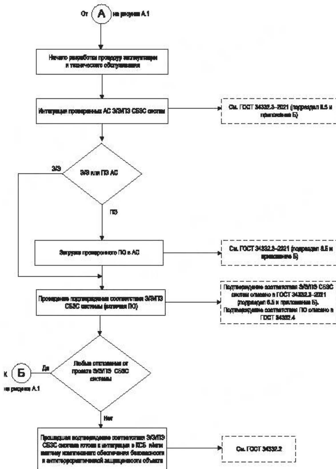
Рисунок А.2 — Функциональные шаги применения ГОСТ 34332.3 (лист 2)
