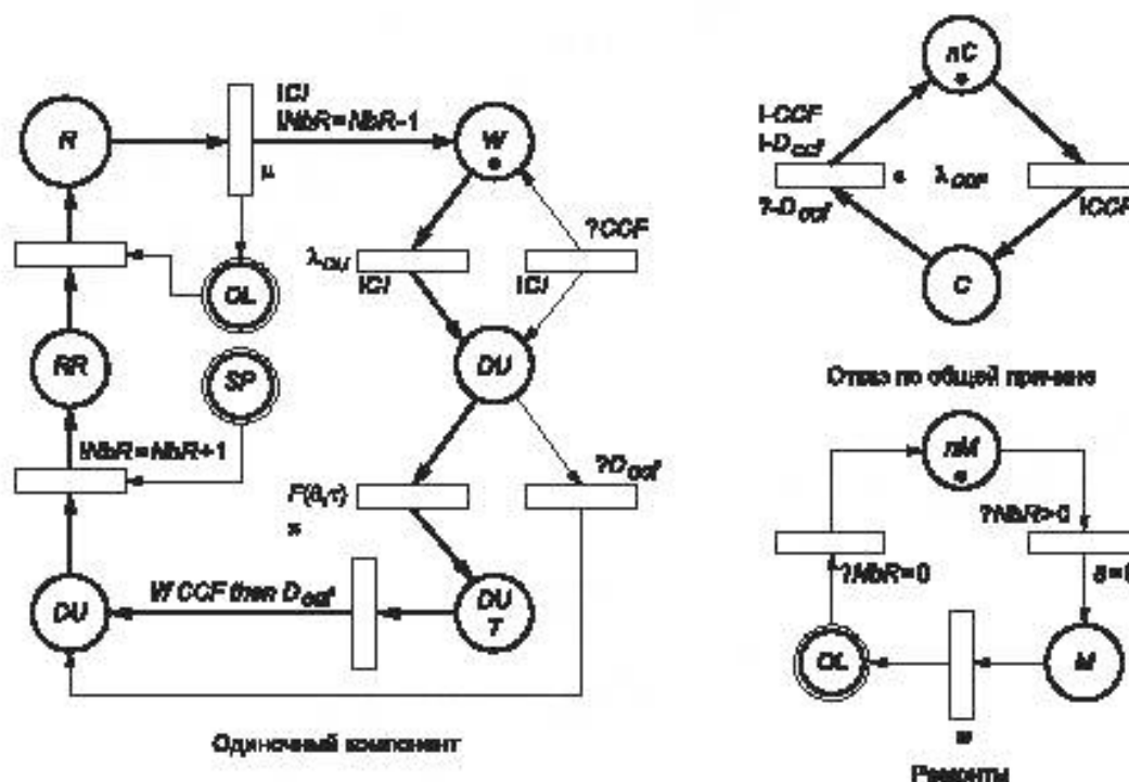
Рисунок Б.34 — Сеть Петри, моделирующая отказ по общей причине и ремонтные ресурсы
