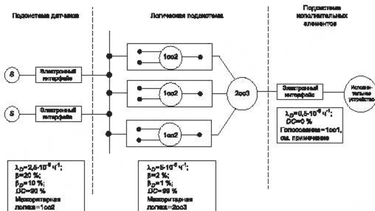
Рисунок Б.15 — Архитектура системы рассматриваемого примера для режима с высокой интенсивностью запросов или с непрерывным запросом
