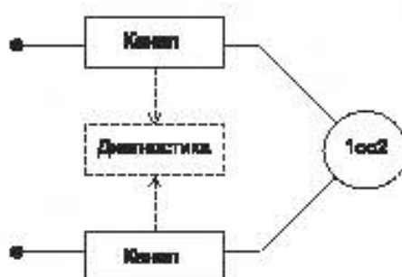
Рисунок Б.6 — Структурная схема архитектуры 1oo2
