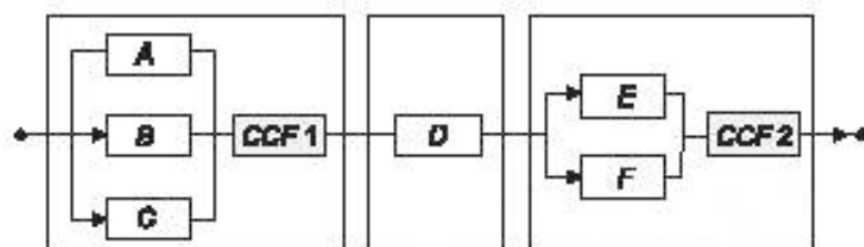
Рисунок Б.1 — Блок-схема надежности полного контура безопасности
