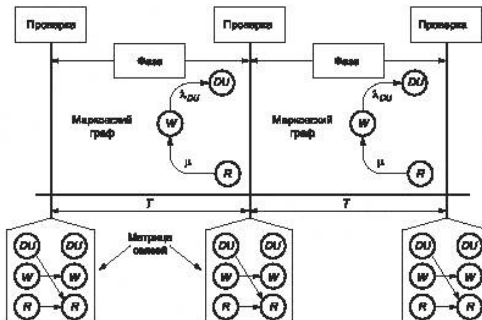
Рисунок Б.24 — Принцип марковского многофазного моделирования
