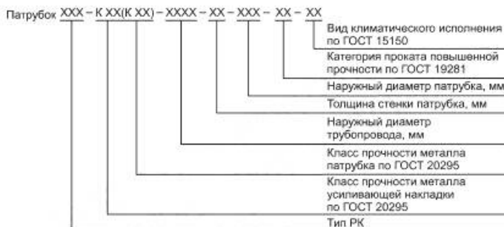
Рисунок 2 — Схема условного обозначения патрубка
