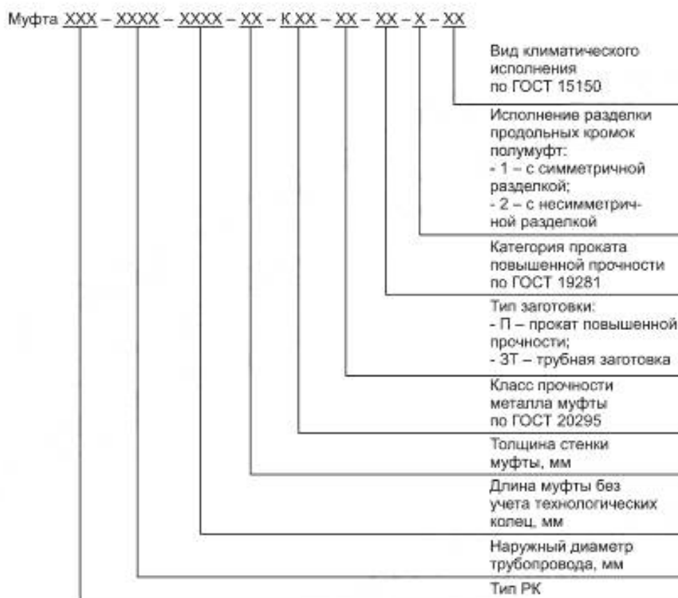
Рисунок 1 — Схема условного обозначения муфты
