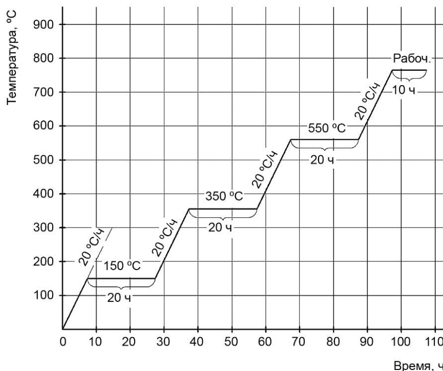
Рисунок 5 — График сушки
