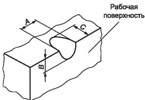
Рисунок 3 — Измерение отбитости ребра
