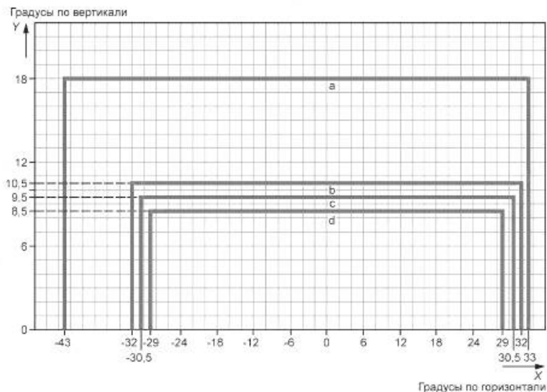
Рисунок Г.17 — Диаграмма изокандел
