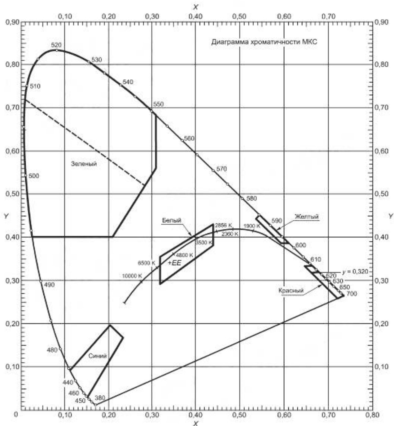
Рисунок И.1 — Диаграмма координат цветности излучения огней
