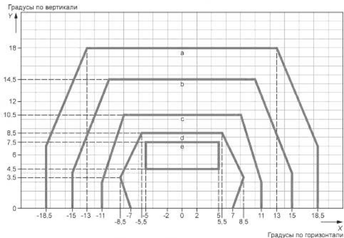
Рисунок Г.18 — Диаграмма изокандел
