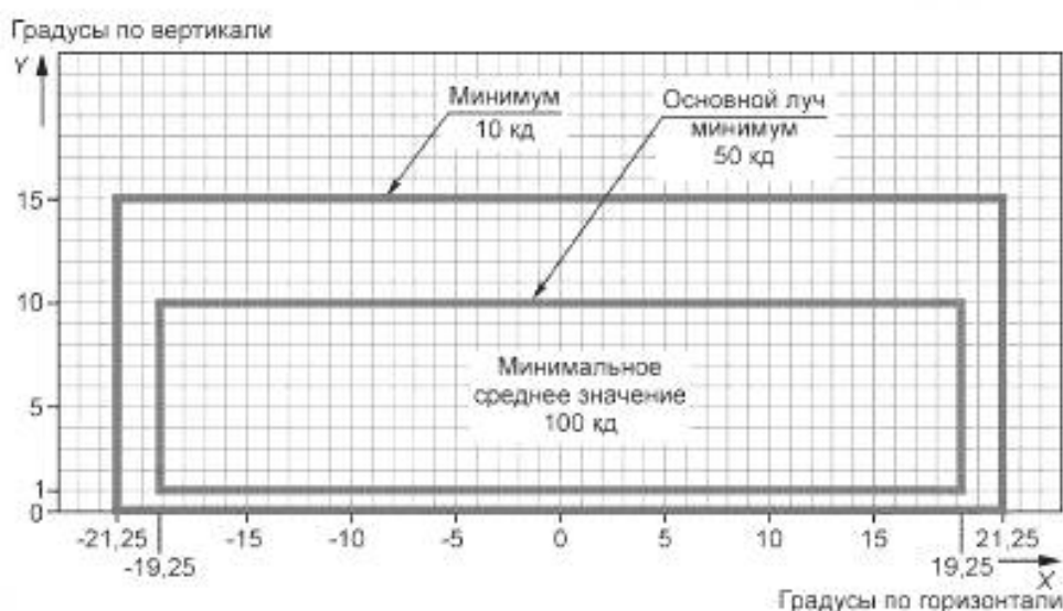
Рисунок Г.13 — Диаграмма изокандел
