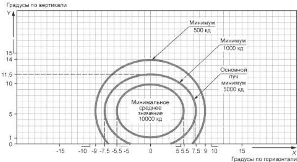
Рисунок Г.3 — Диаграмма изокандел
