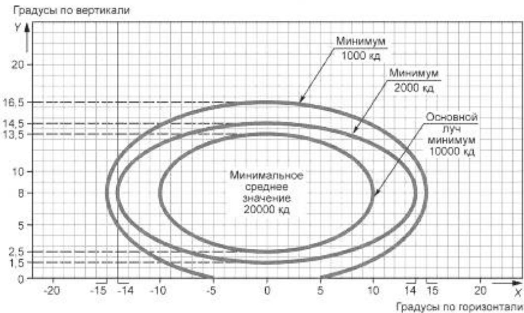
Рисунок Г.1 — Диаграмма изокандел
