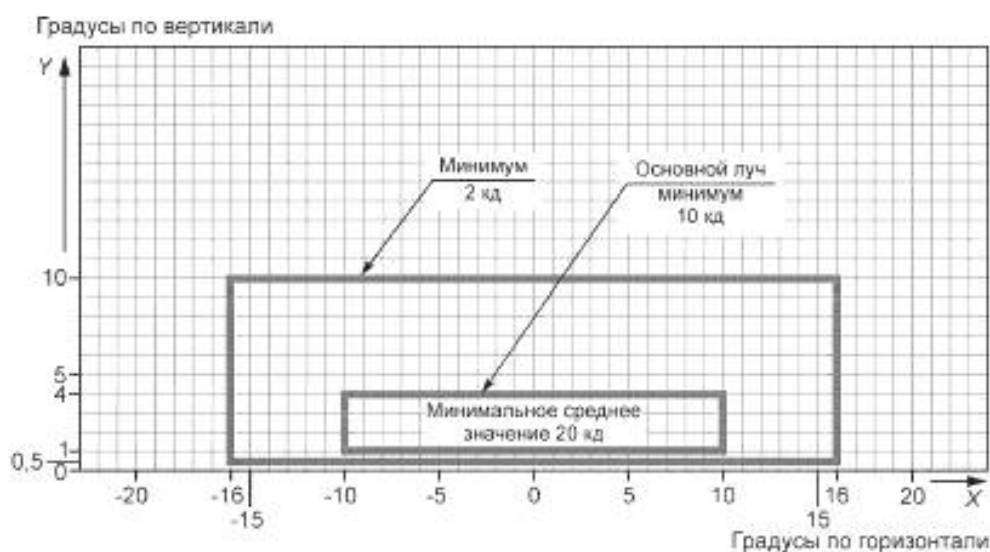
Рисунок Г.14 — Диаграмма изокандел
