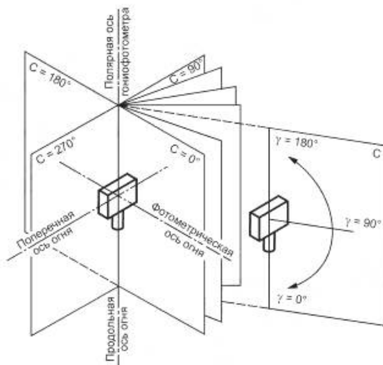
Рисунок В.1 — Система фотометрирования C, \gamma
