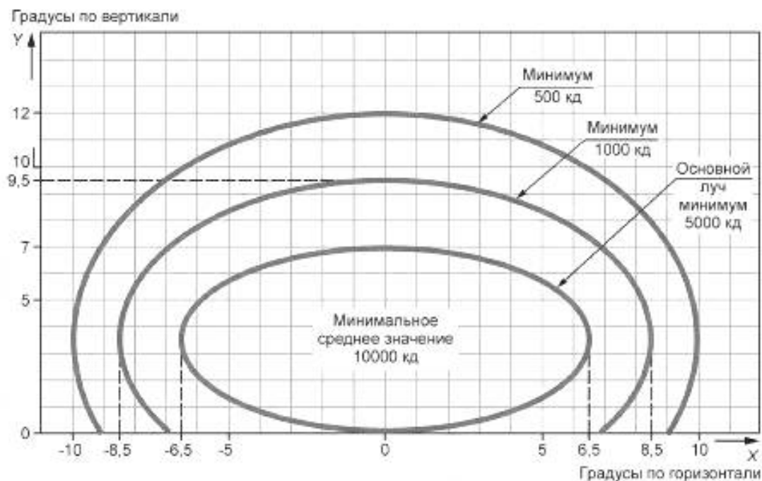
Рисунок Г.10 — Диаграмма изокандел
