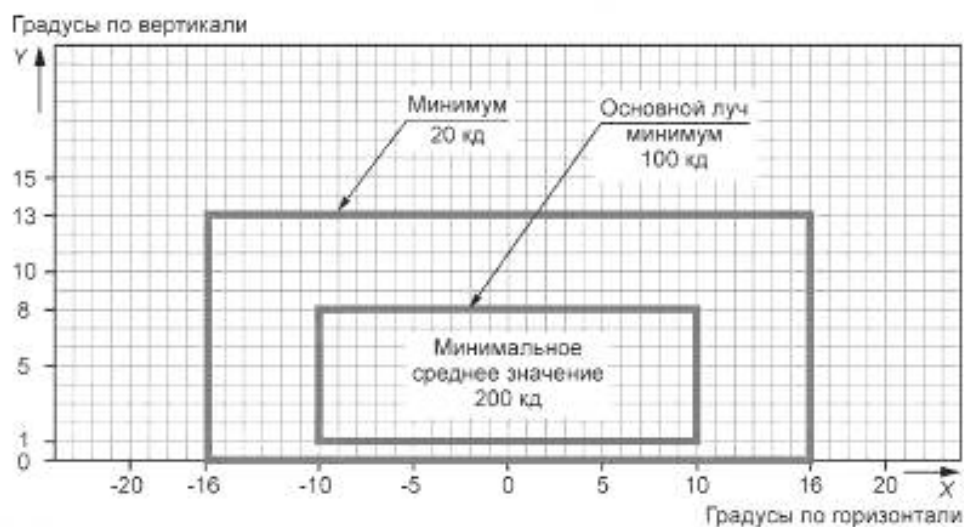
Рисунок Г.11 — Диаграмма изокандел
