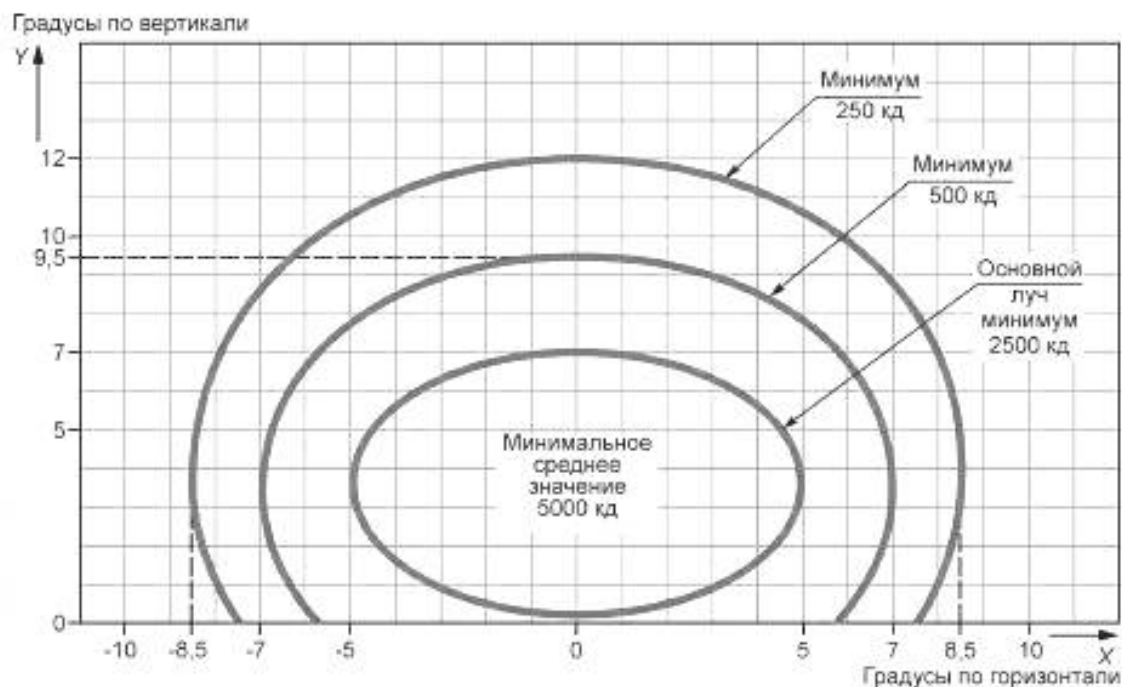
Рисунок Г.6 — Диаграмма изокандел
