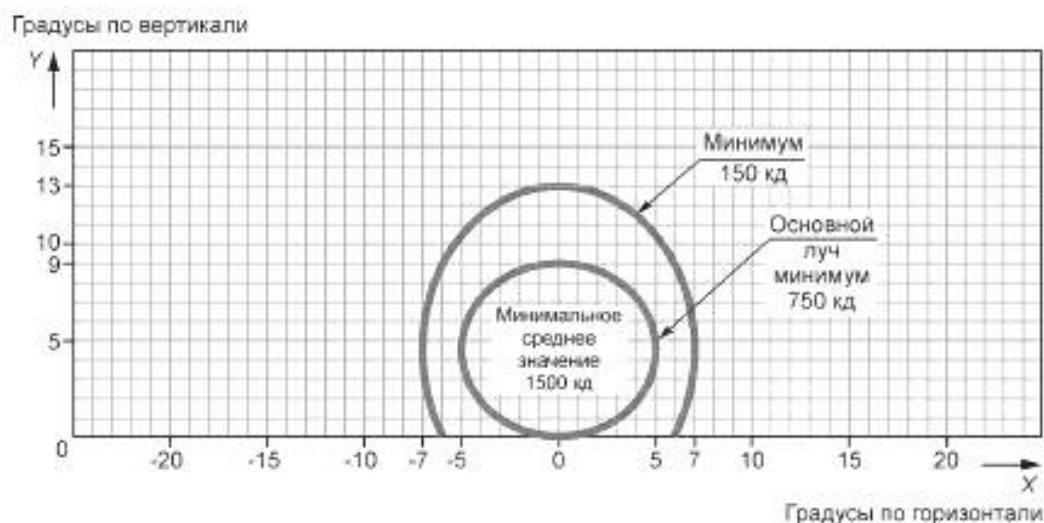
Рисунок Г.19 — Диаграмма изокандел
