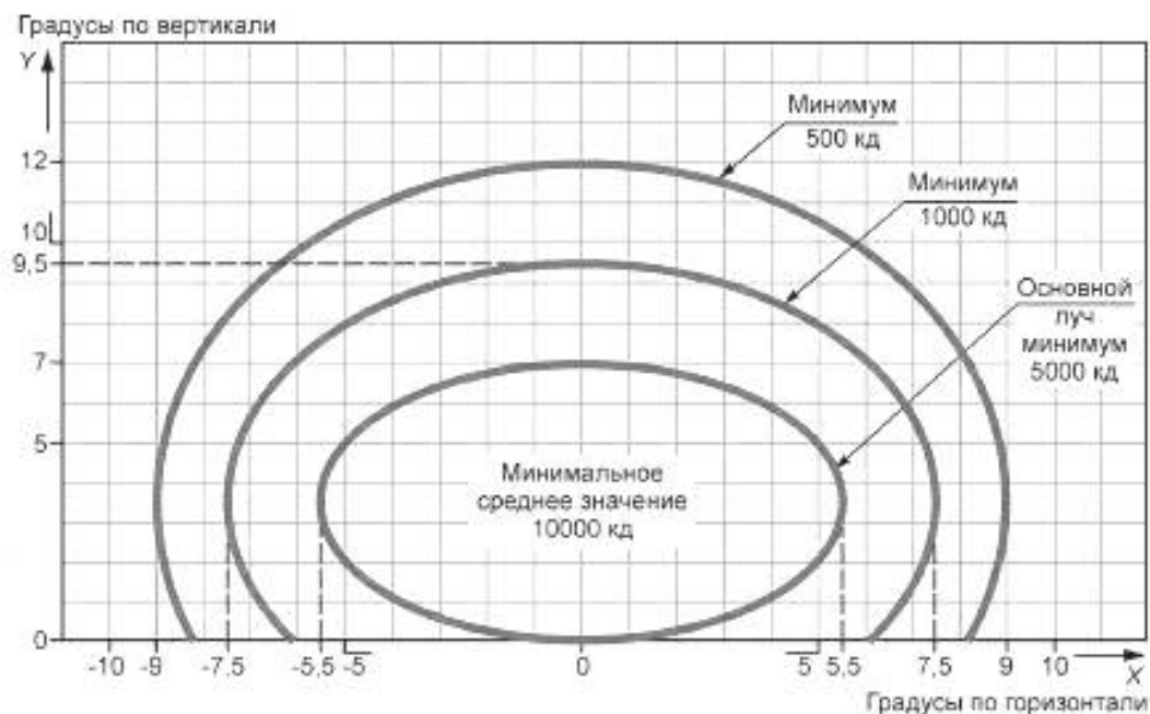
Рисунок Г.9 — Диаграмма изокандел
