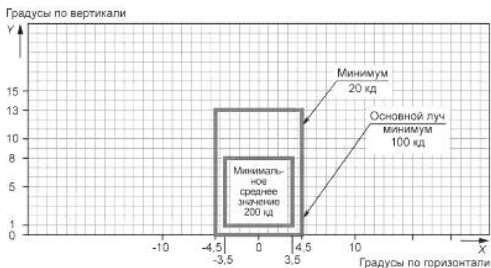
Рисунок Г.12 — Диаграмма изокандел
