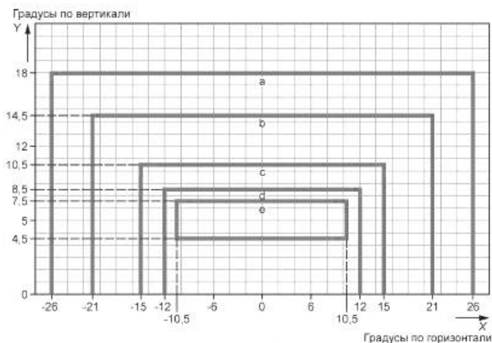
Рисунок Г.16 — Диаграмма изокандел
