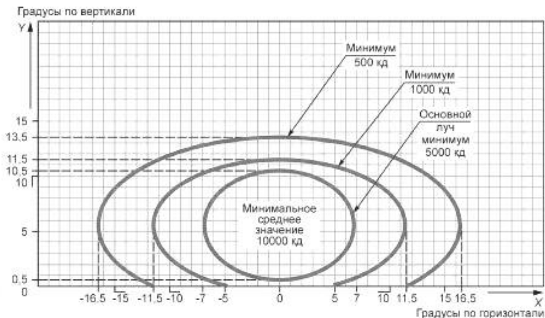
Рисунок Г.4 — Диаграмма изокандел
