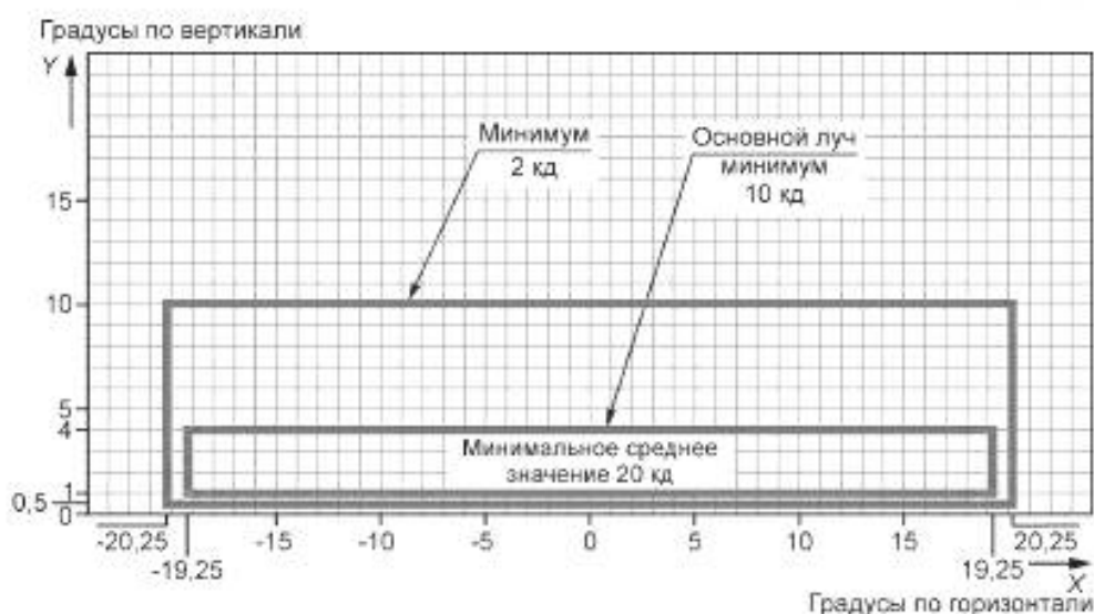
Рисунок Г.15 — Диаграмма изокандел
