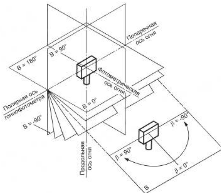
Рисунок В.2 — Система фотометрирования B, \beta
