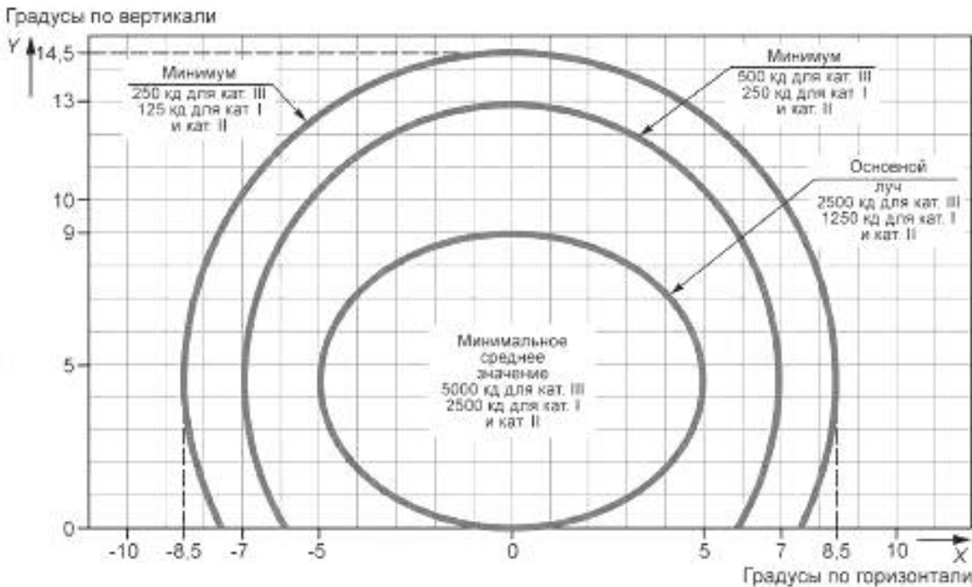
Рисунок Г.7 — Диаграмма изокандел
