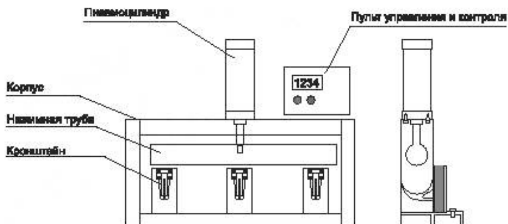
Рисунок 7 — Схема испытательного стенда кронштейнов
