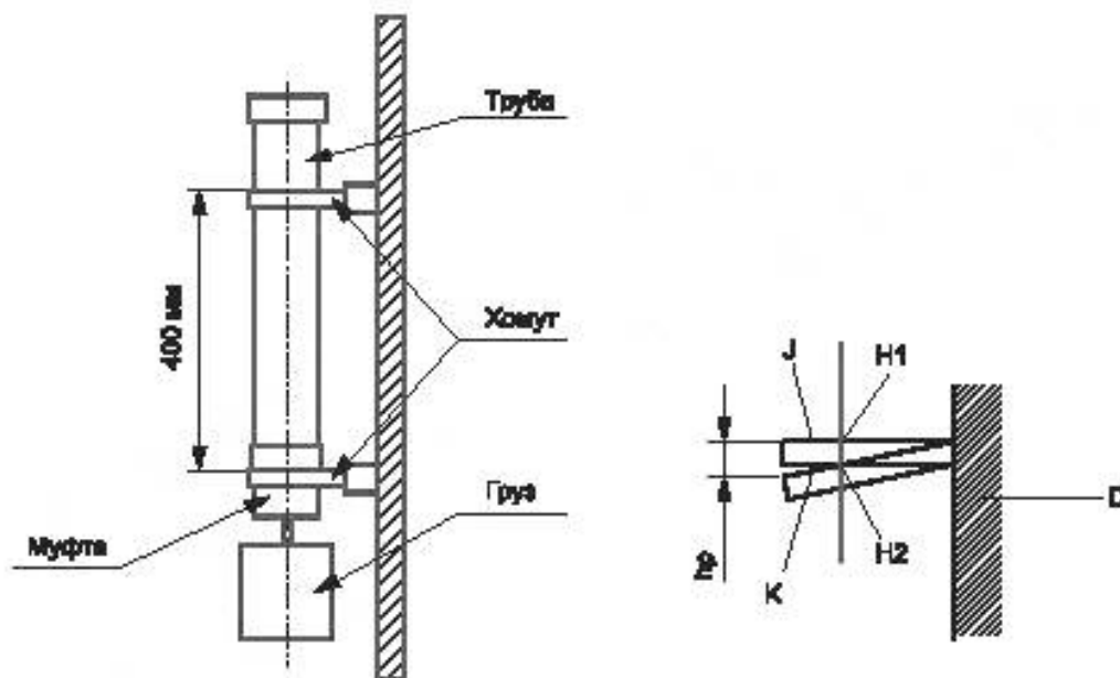
Рисунок 5 — Схема испытания хомутов на сопротивление внешним воздействиям
