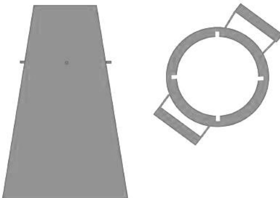
Рисунок А.1 — Схема конуса со съемными ручками для определения удобоукладываемости серобетонной смеси.
