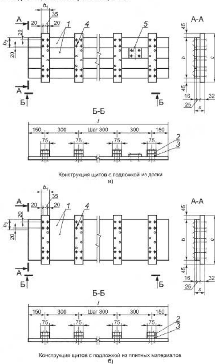
Рисунок А.1 — Конструкция и основные размеры щита
