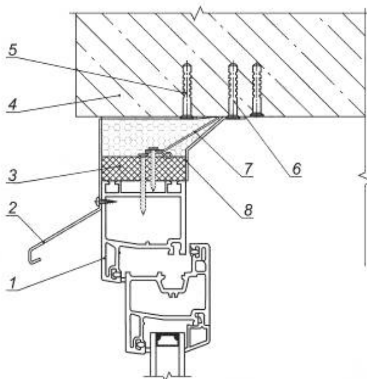
1 — оконный блок; 2 — козырек; 3 — теплоизоляционный вкладыш; 4 — балконная плита; 5 — элемент крепления козырька; 6 — элемент крепления анкерной пластины; 7 — пластина анкерная; 8 — пароизоляция
