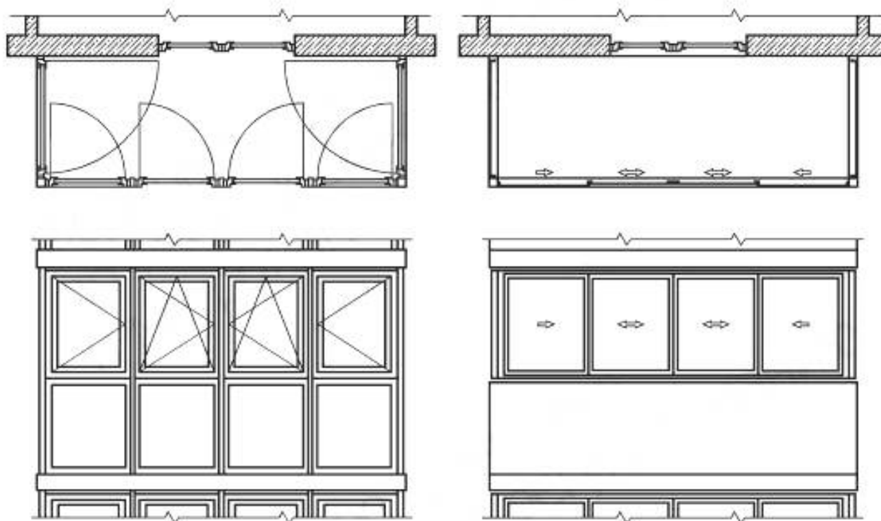
Рисунок Б.7 — Примеры конструкций наружного остекления
