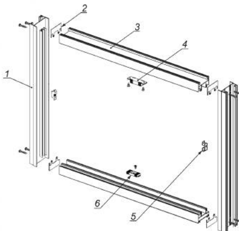
1 — профиль рамы вертикальный; 2 — прокладка торца рамы; 3 — профиль рамы горизонтальный; 4 — верхний уплотнитель створки; 5 — ответная часть защелки; 6 — нижний уплотнитель створки
