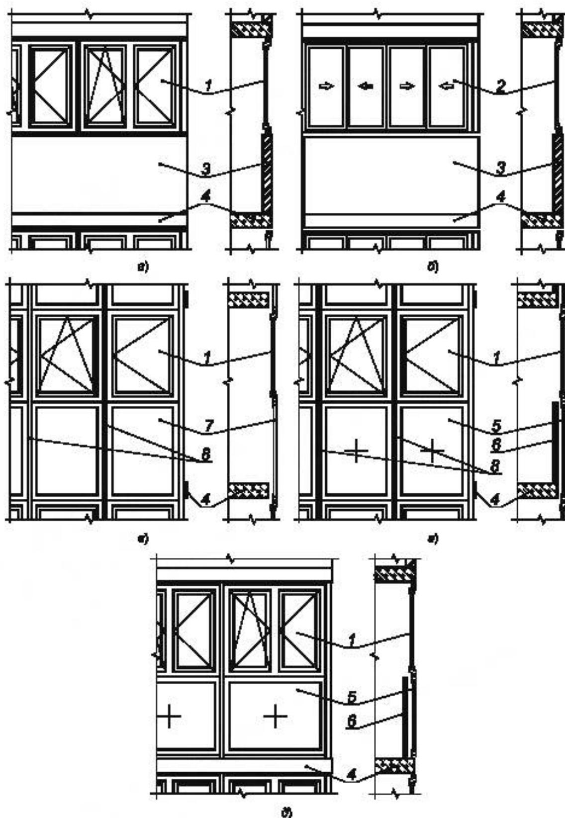
а) — балкон с ленточным остеклением; б) — балкон с раздвижным остеклением; в) — стоечное ограждение балкона с непрозрачным заполнением; г) — стоечное ограждение балкона с панорамным остеклением; д) — балкон с панорамным остеклением
