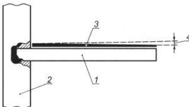
Рисунок Б.2 — Выполнение уклона цементной стяжки на балконной плите
