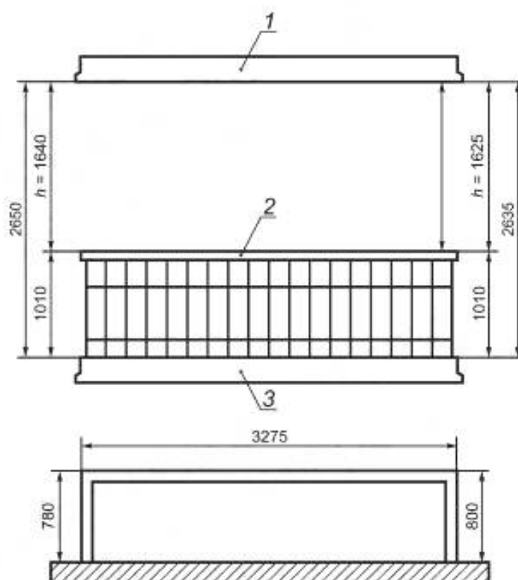
1, 3 — железобетонная плита балкона; 2 — ограждающий поручень
