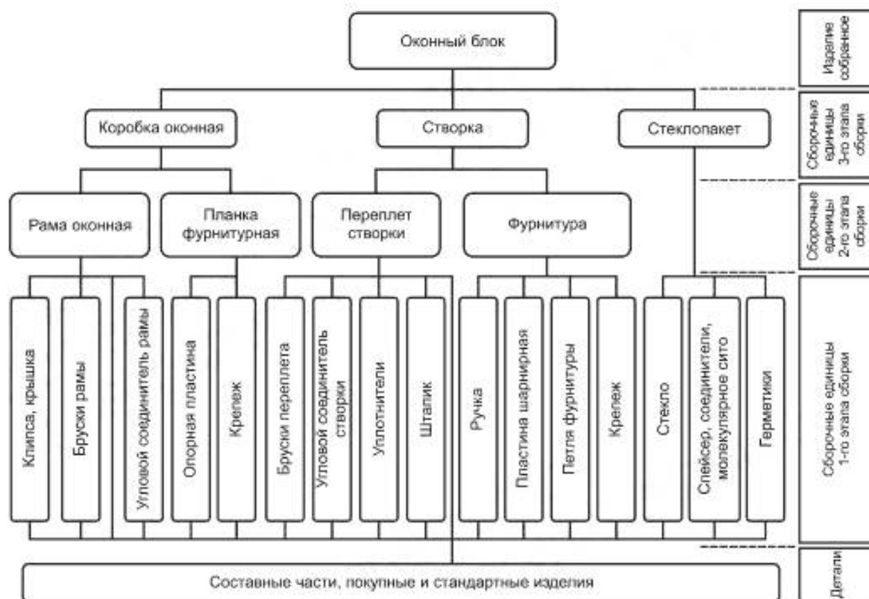
Рисунок А.4 — Схема сборки оконного блока
