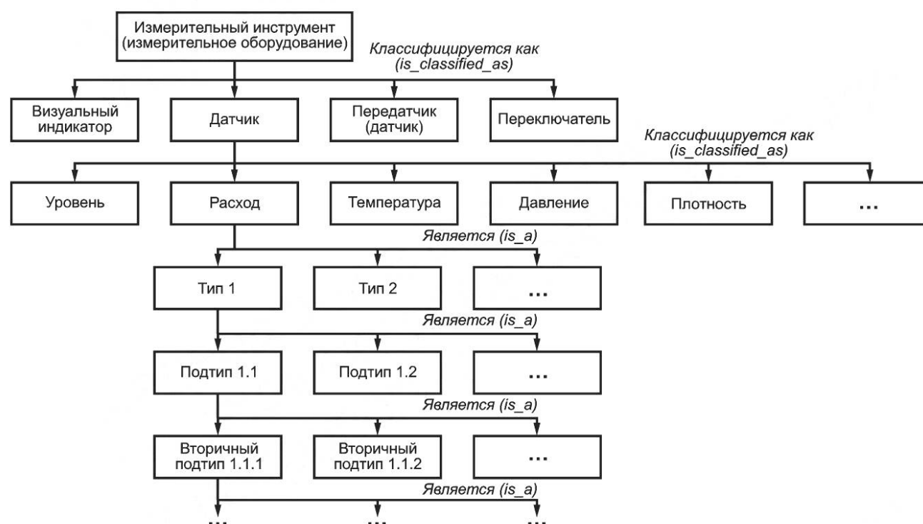
Рисунок 1 — Классификационная схема измерительного оборудования
