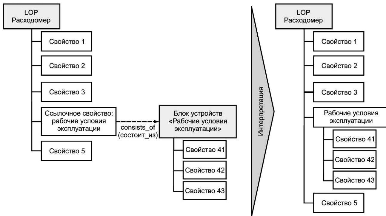
Рисунок 4 — Содержимое блока свойств
