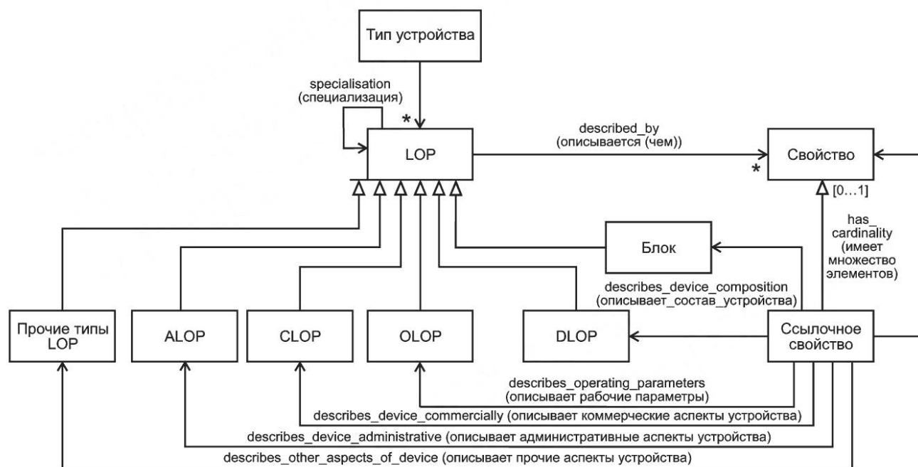
Рисунок А.1 — Упрощенная схема UML перечней свойств
