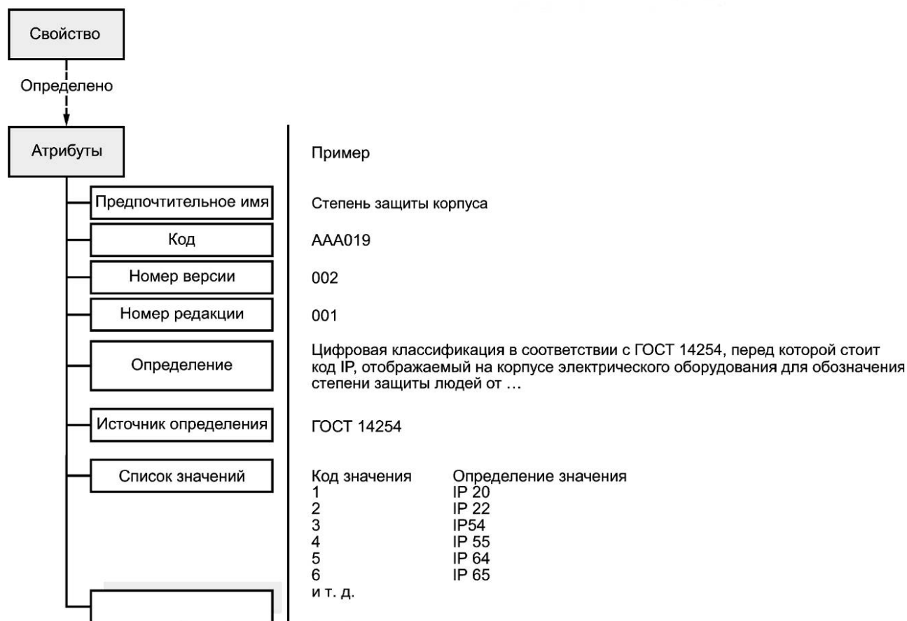
Рисунок 3 — Свойство и его атрибуты
