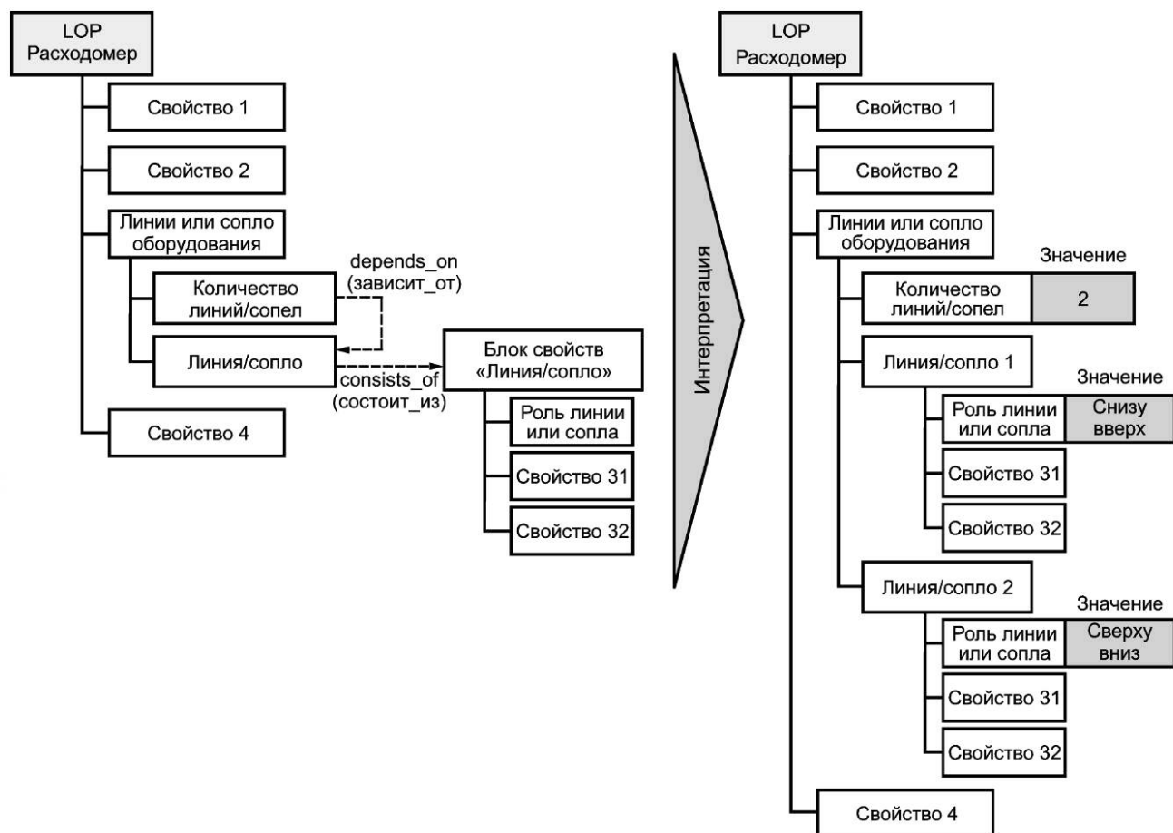
Рисунок 5 — Пример множества элементов
