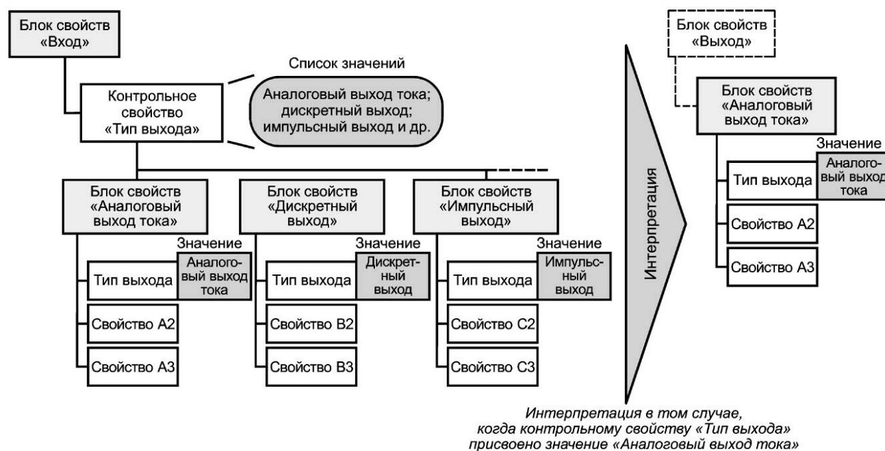
Рисунок 6 — Пример полиморфизма
