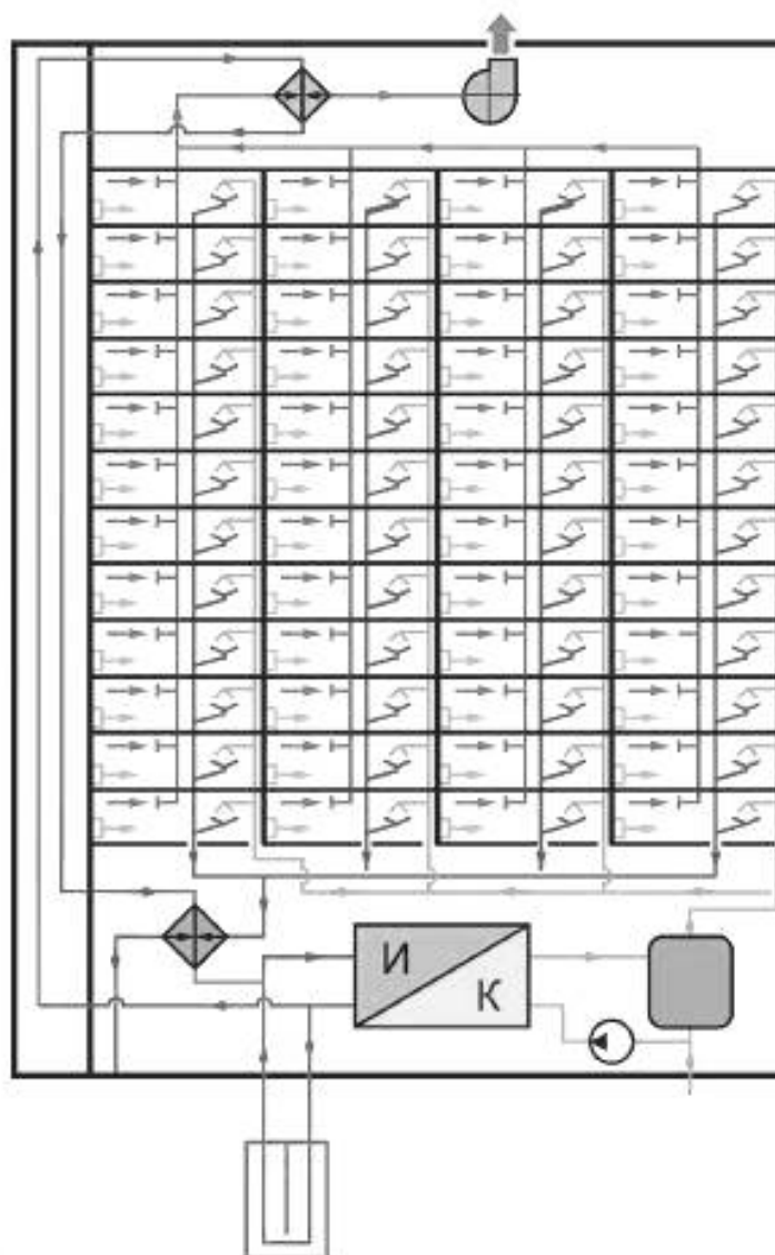
Рисунок 9 — Комбинированное использование теплоты вентиляционных выбросов, грунта и канализационных стоков жилого дома
