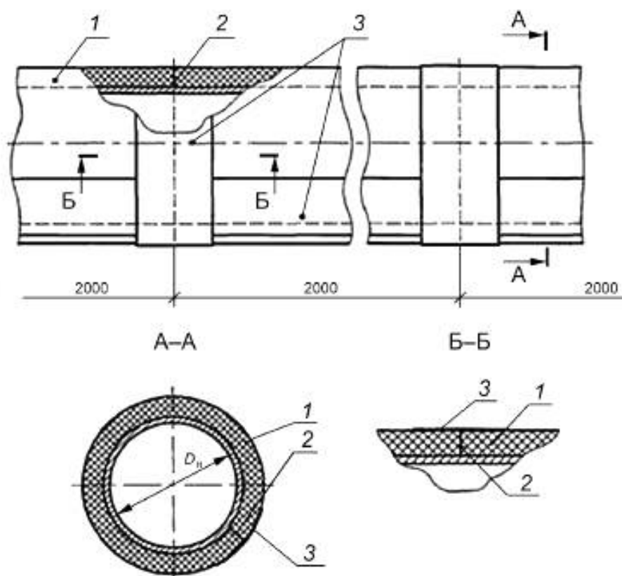
Рисунок 1 — Теплоизоляционная конструкция трубопровода диаметром D_n
