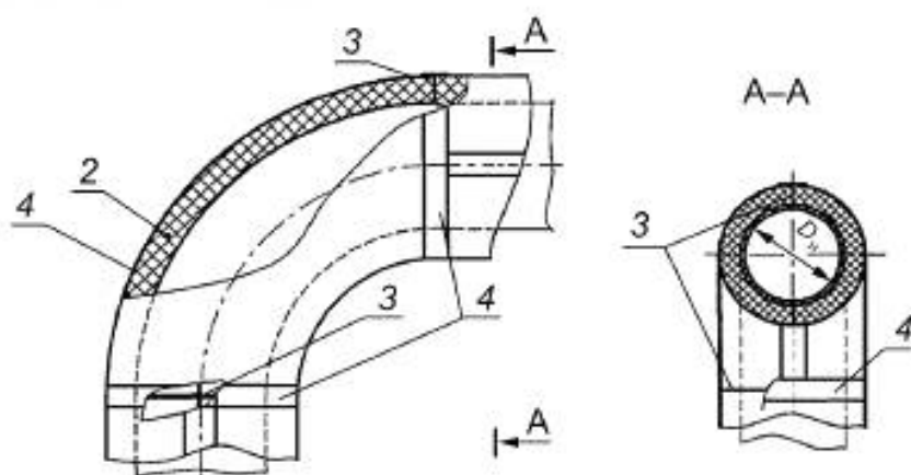
б) Изоляция отвода термоизоляционными листами ( D_{\text{н}} > 160 мм)
