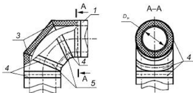
а) Изоляция отвода термоизоляционными трубками ( D_{\text{н}} \leq 160 мм)
