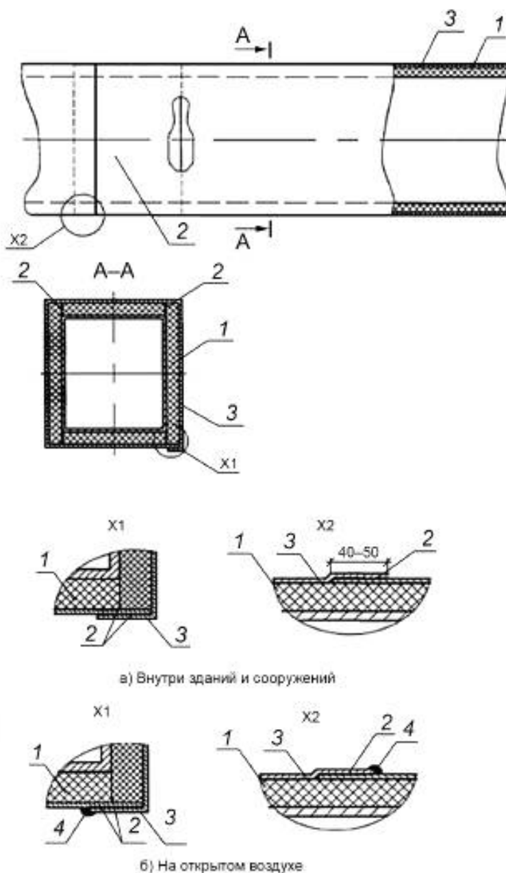
Рисунок 10 — Теплоизоляционная конструкция воздуховода с металлической оболочкой
